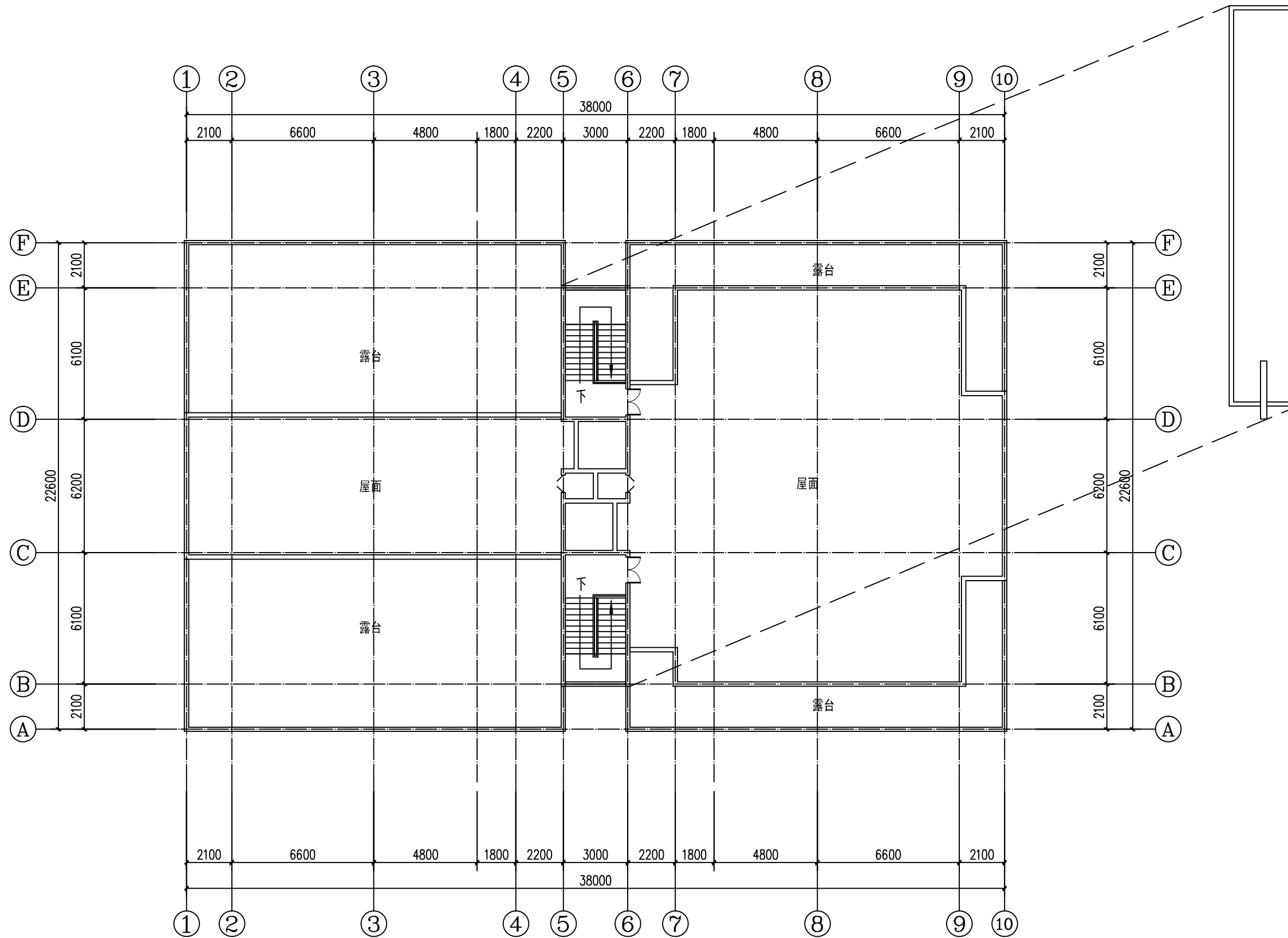
屋面层平面图
