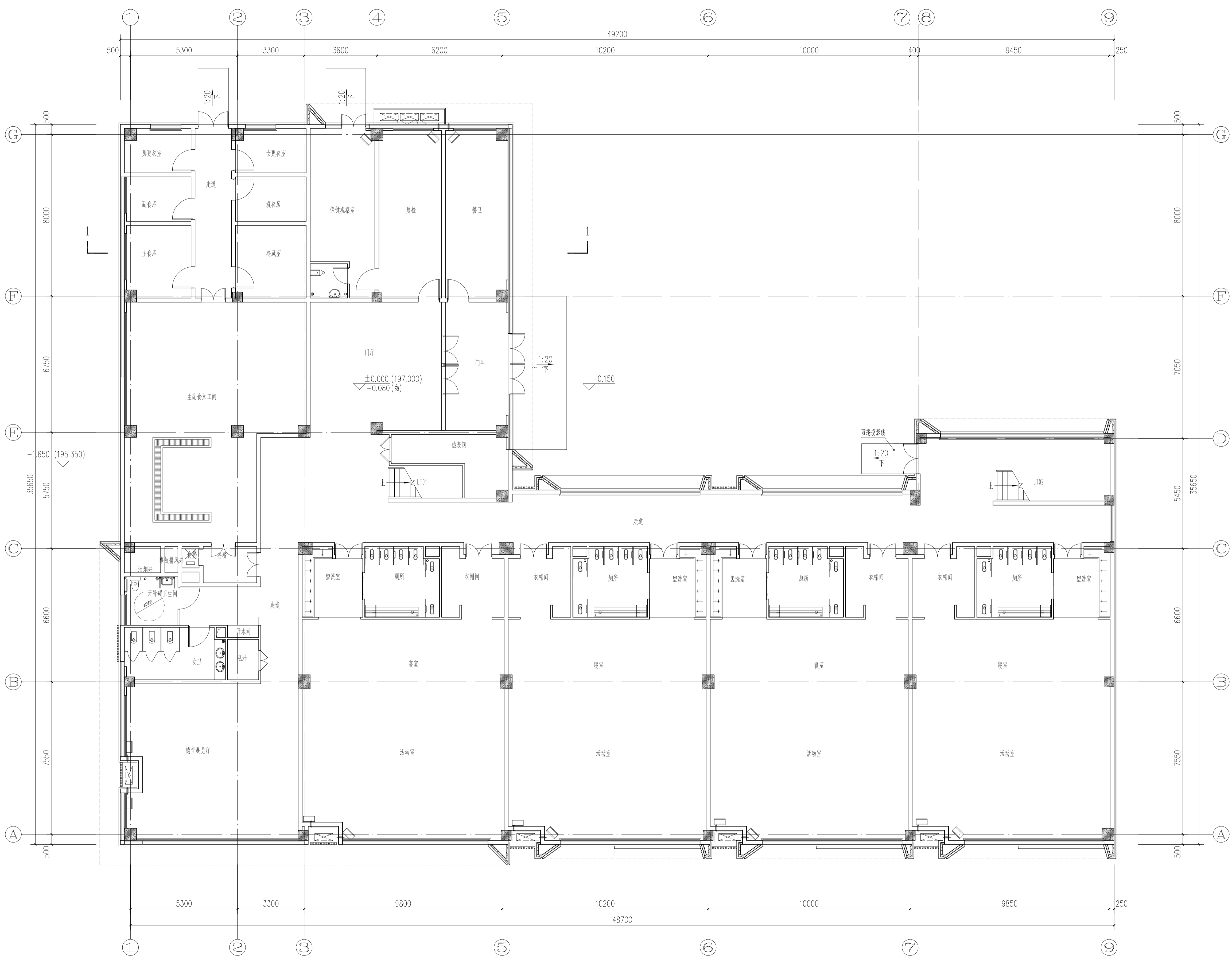
一层平面图 1:100
