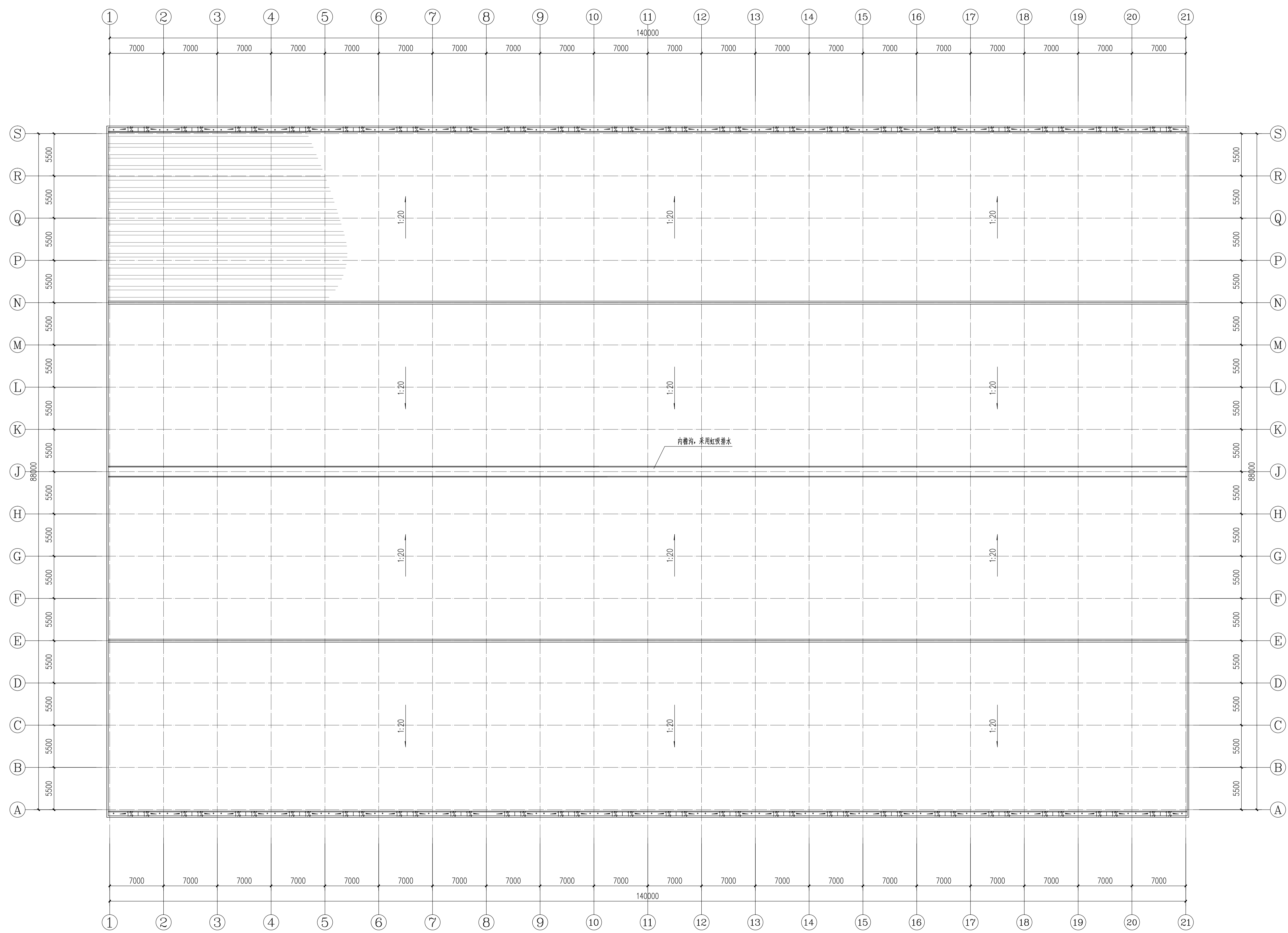
屋顶平面图 1:250
