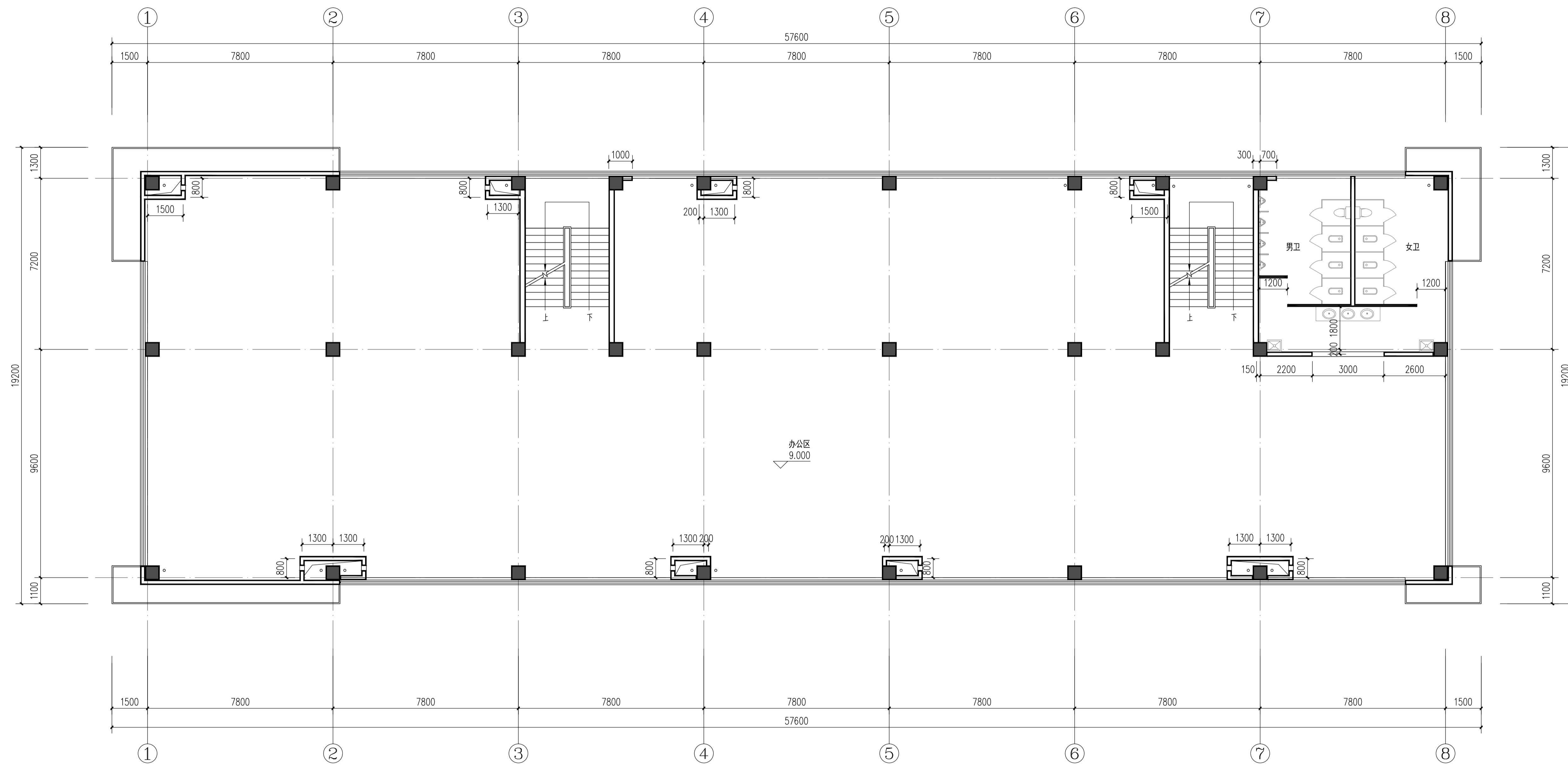
三层平面图 1:100 本层建筑面积:994.56m 2
