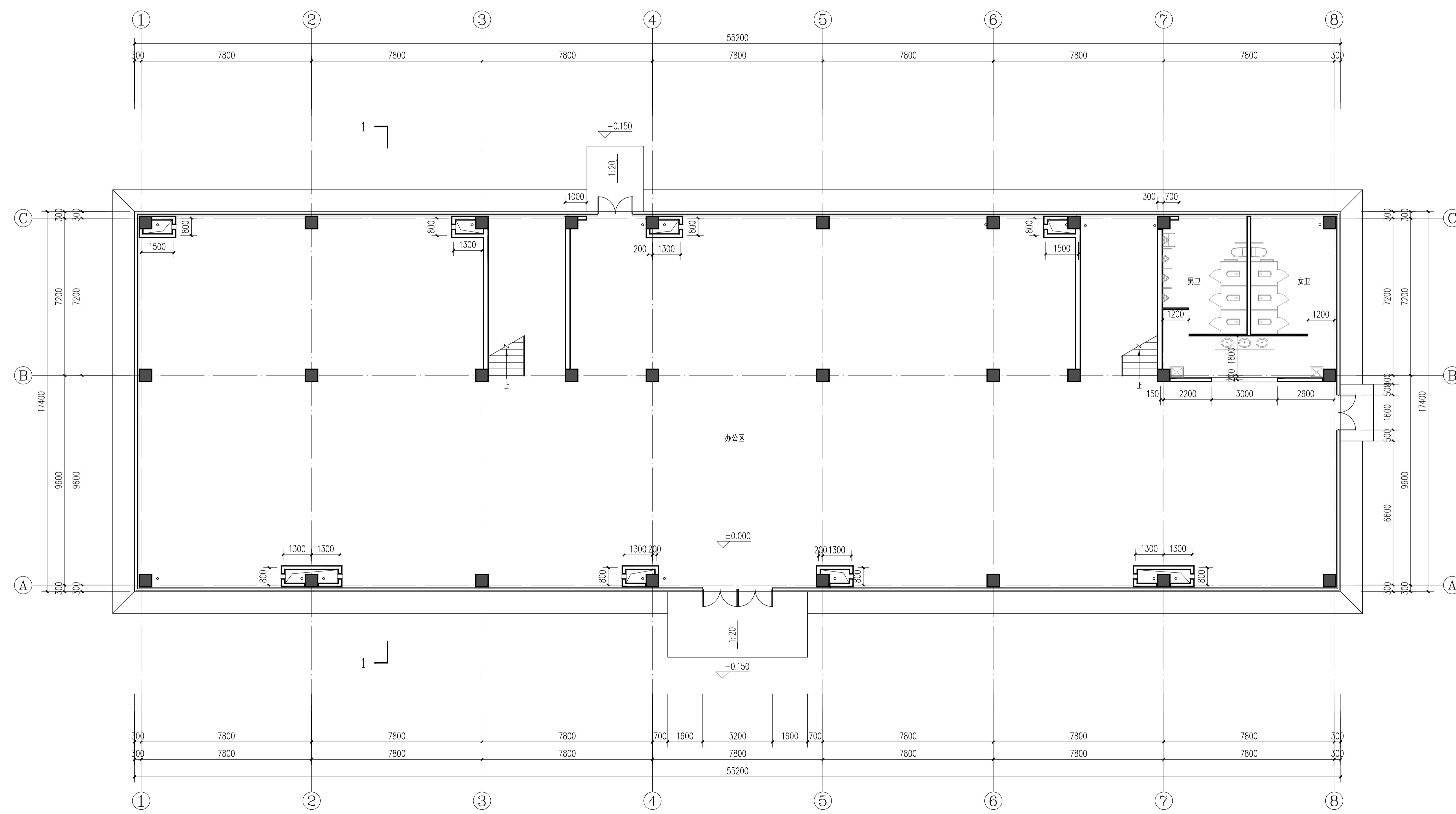
一层平面图 1:100
