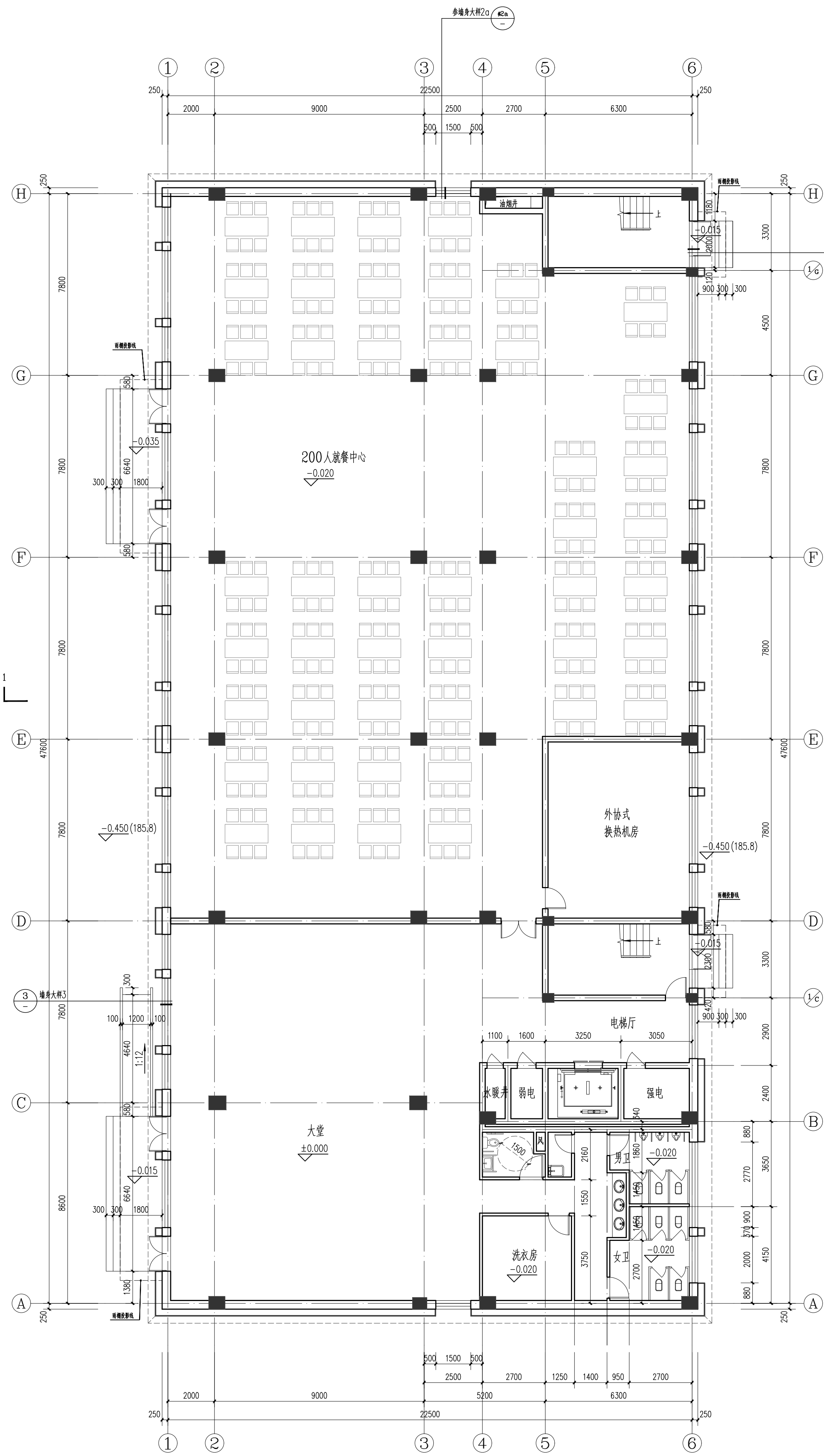
一层平面图 1:100
