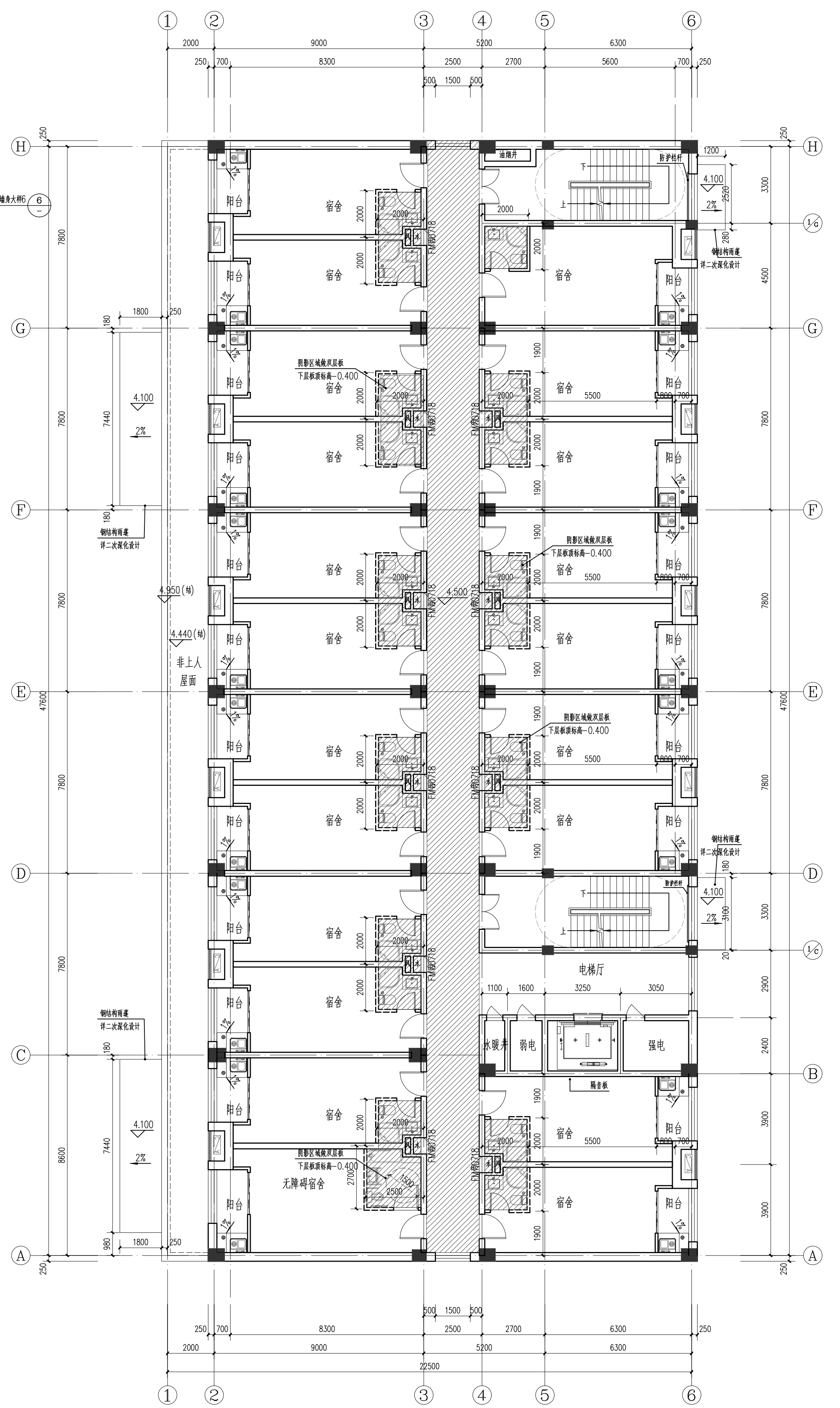
二层平面图 1:100
