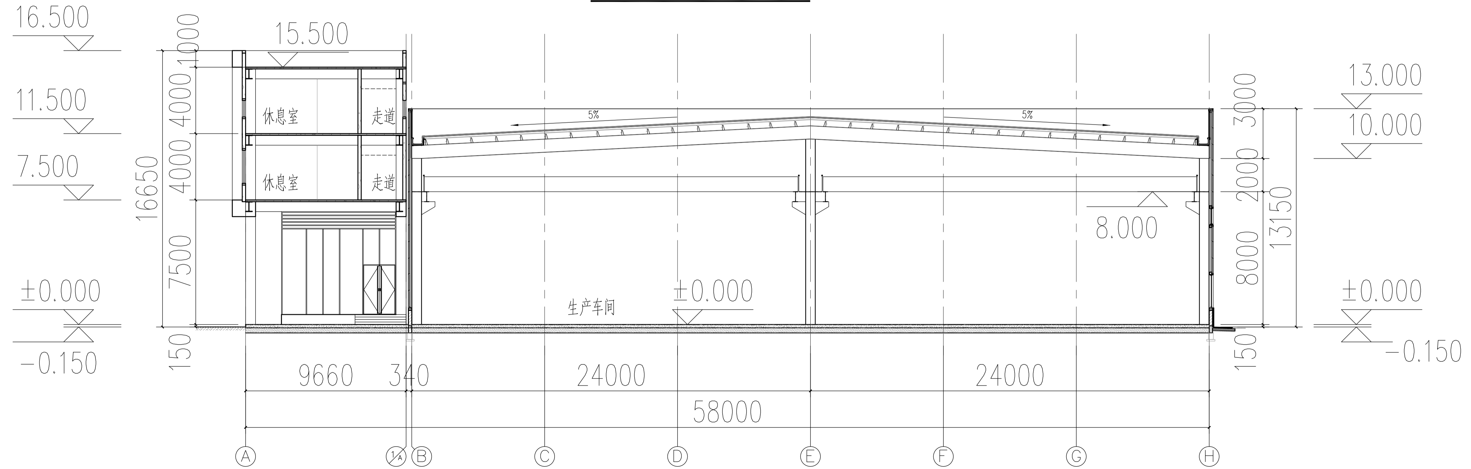
1号厂房2-2剖面图 1:150
