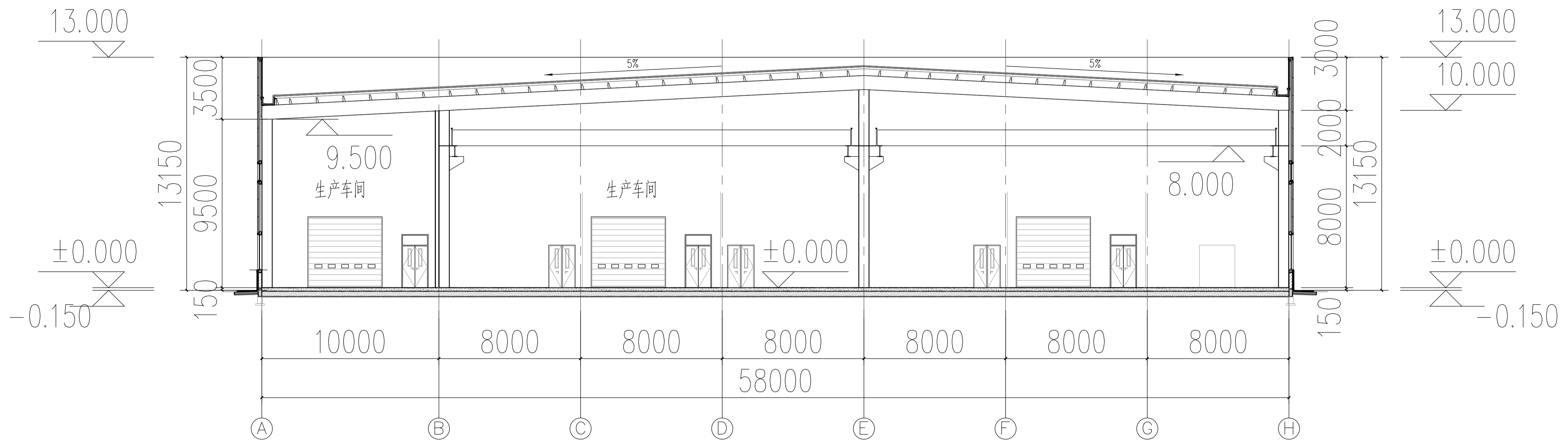
1号厂房1-1剖面图 1:150
