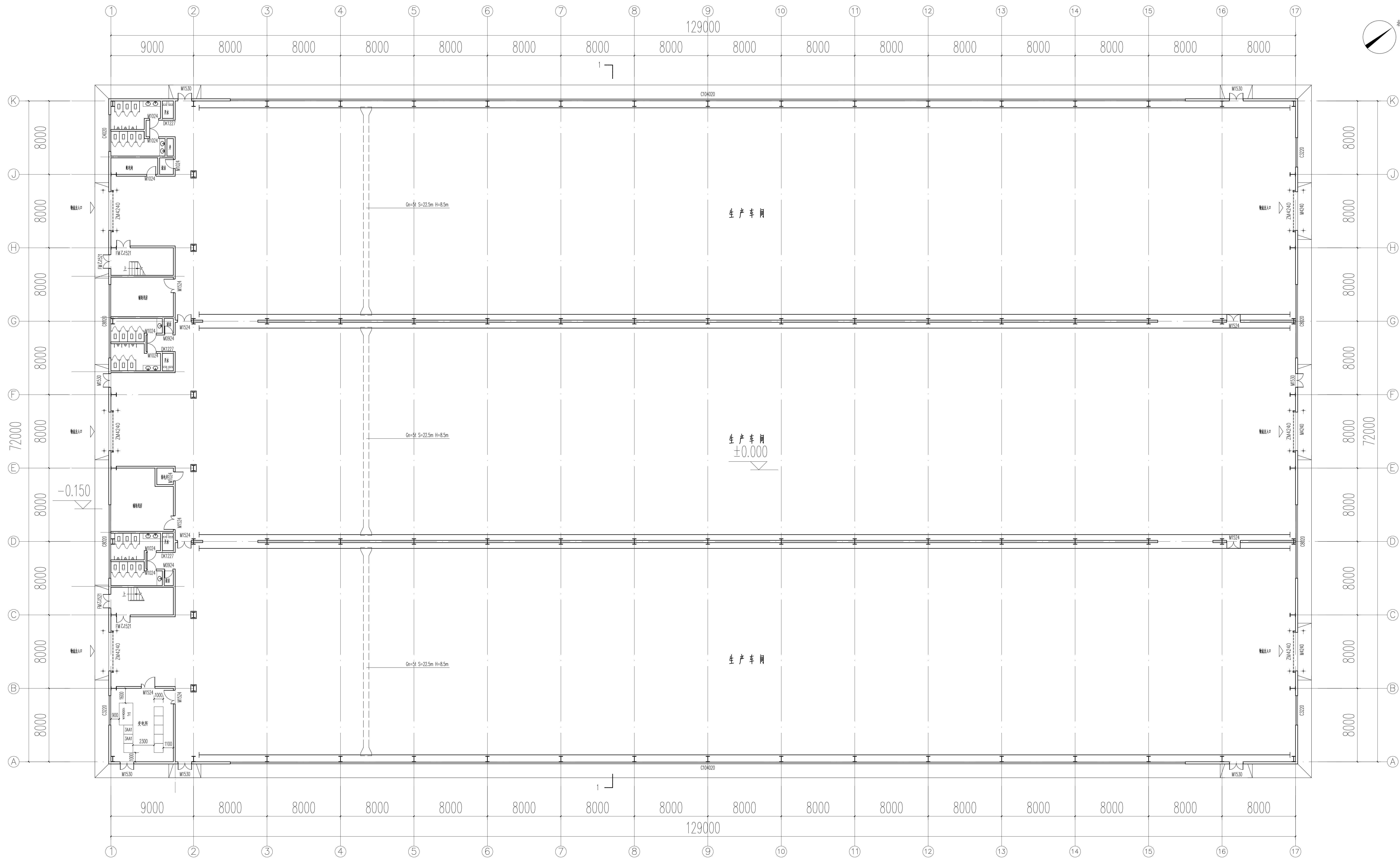
2号厂房一层平面图 本层建筑面积9384.71平方米 总建筑面积10083.42平方米
