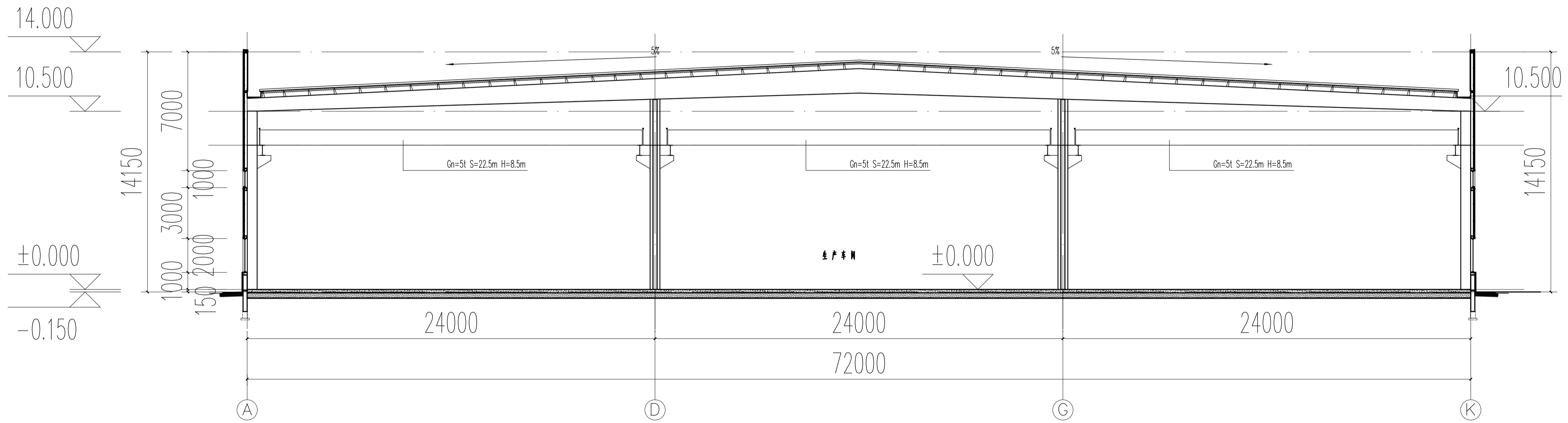
2号厂房 1-1剖面图
