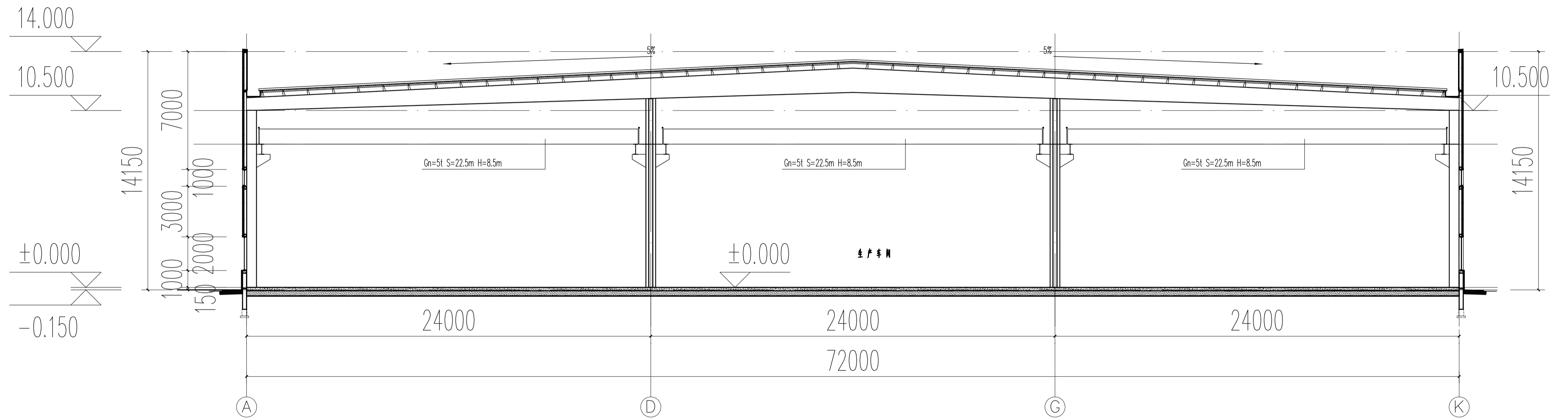
3号厂房 1-1剖面图
