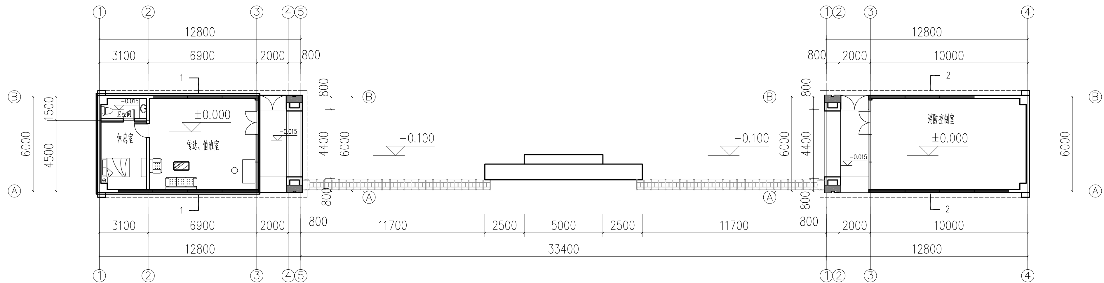
一层平面图 1:100
