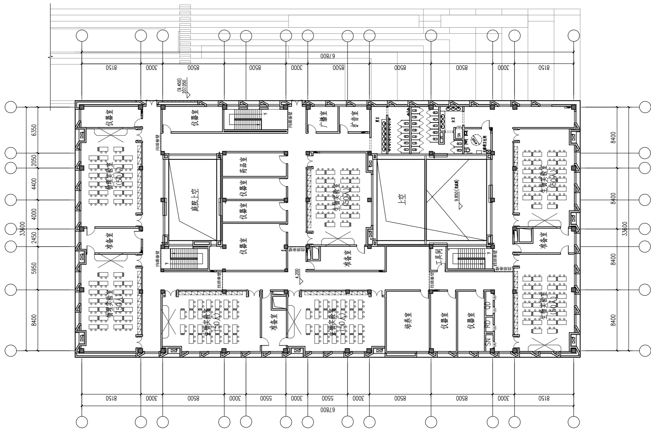
二层平面图
