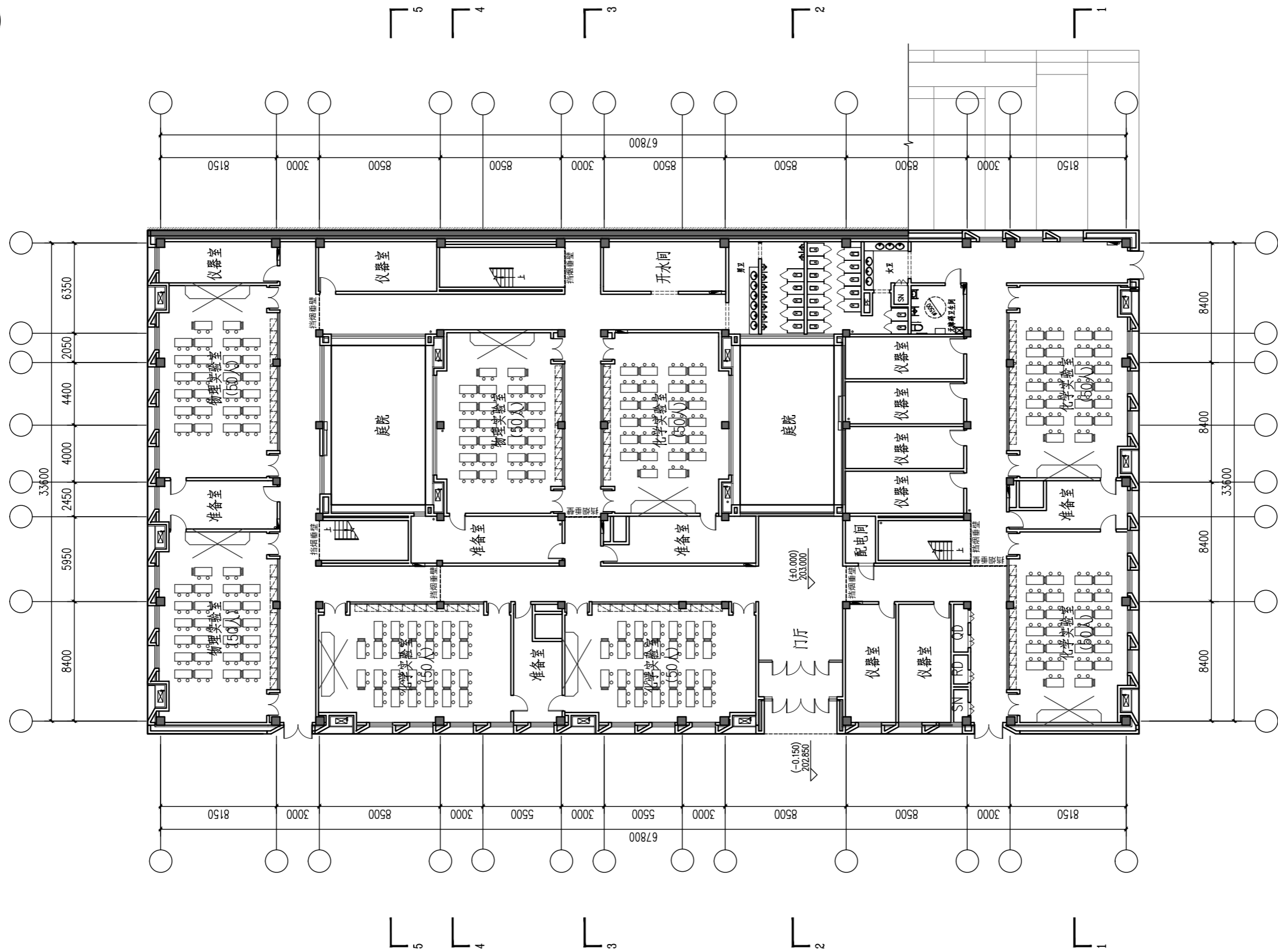
首层平面图
