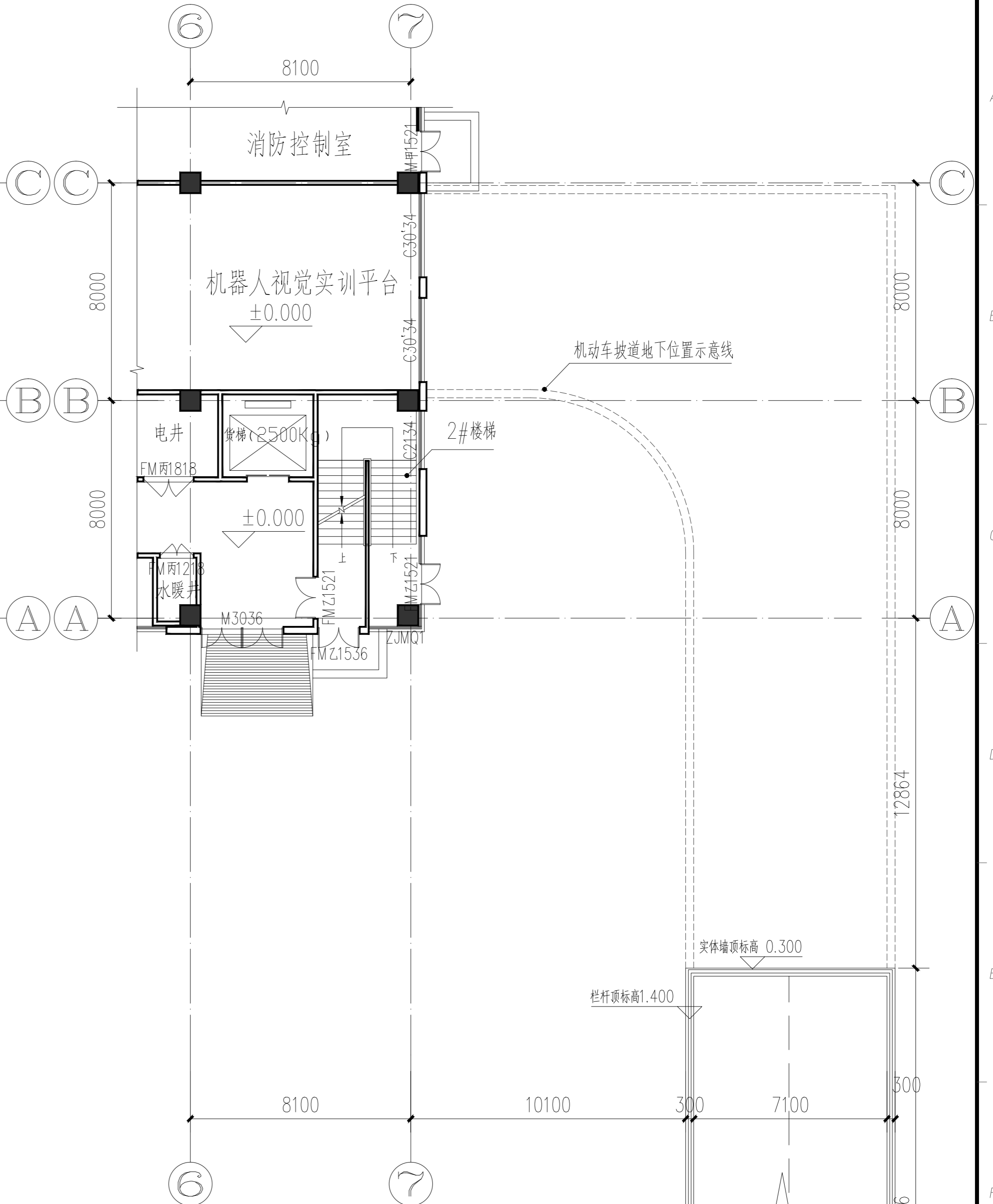
机动车坡道一层平面图 1:120
