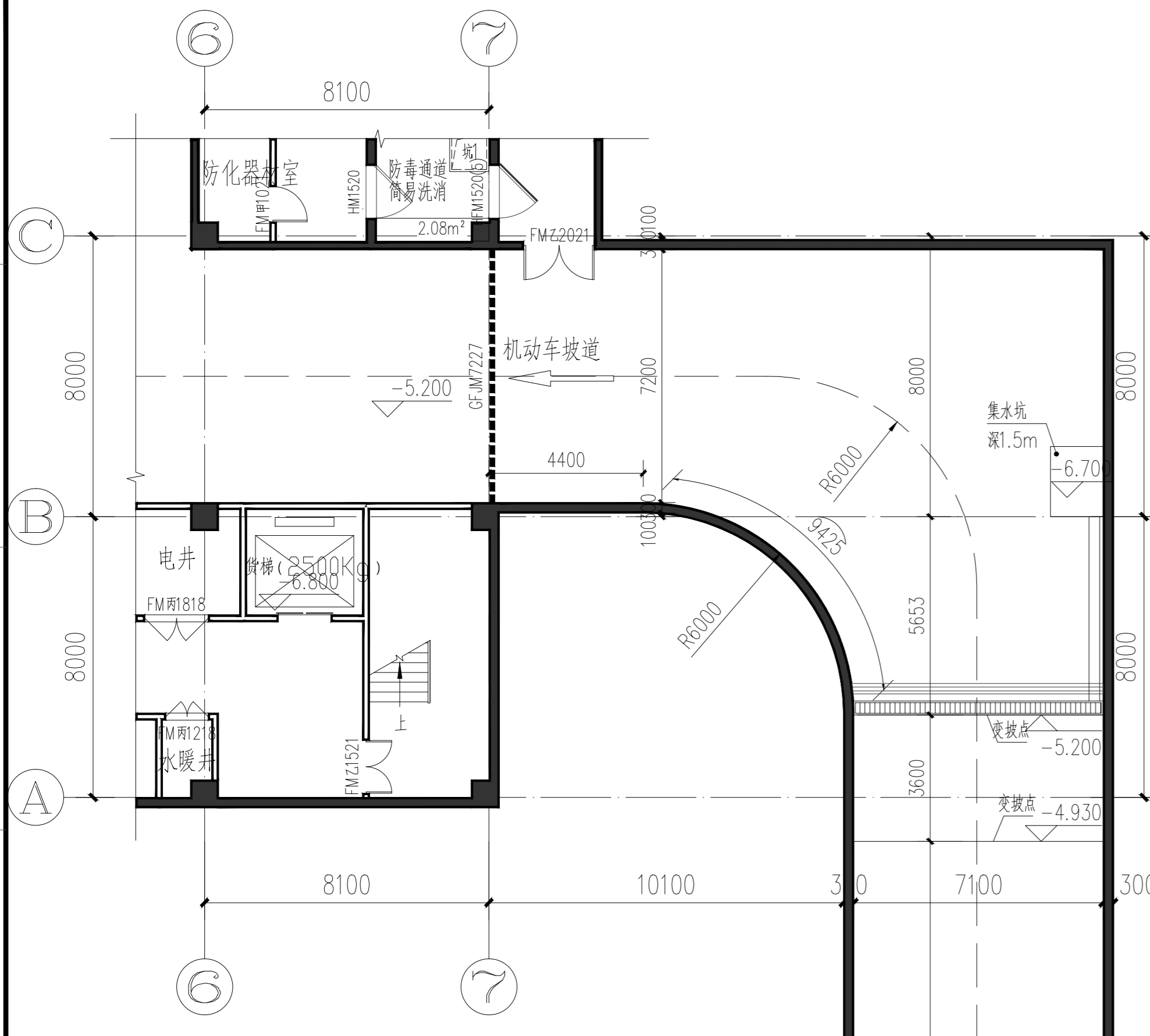
机动车坡道下一层平面图 1:120
