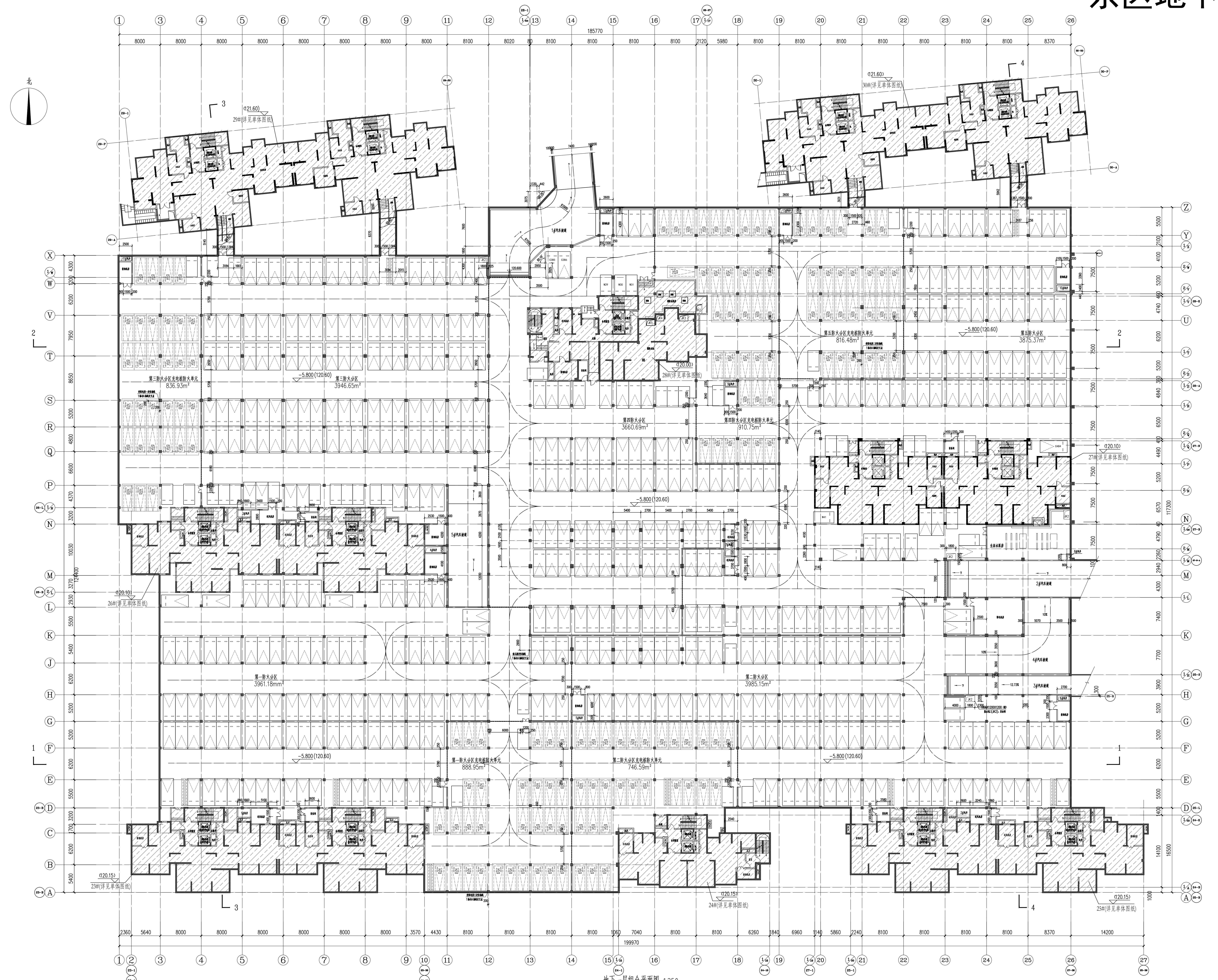
地下一层组合平面图 1:200
