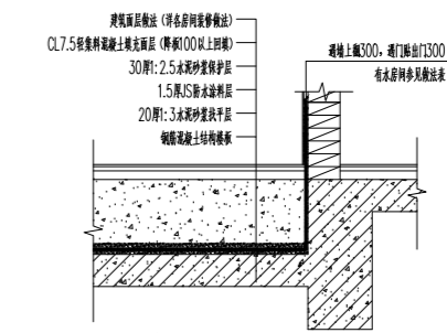
1 降板区同层防水回填做法 1:20
