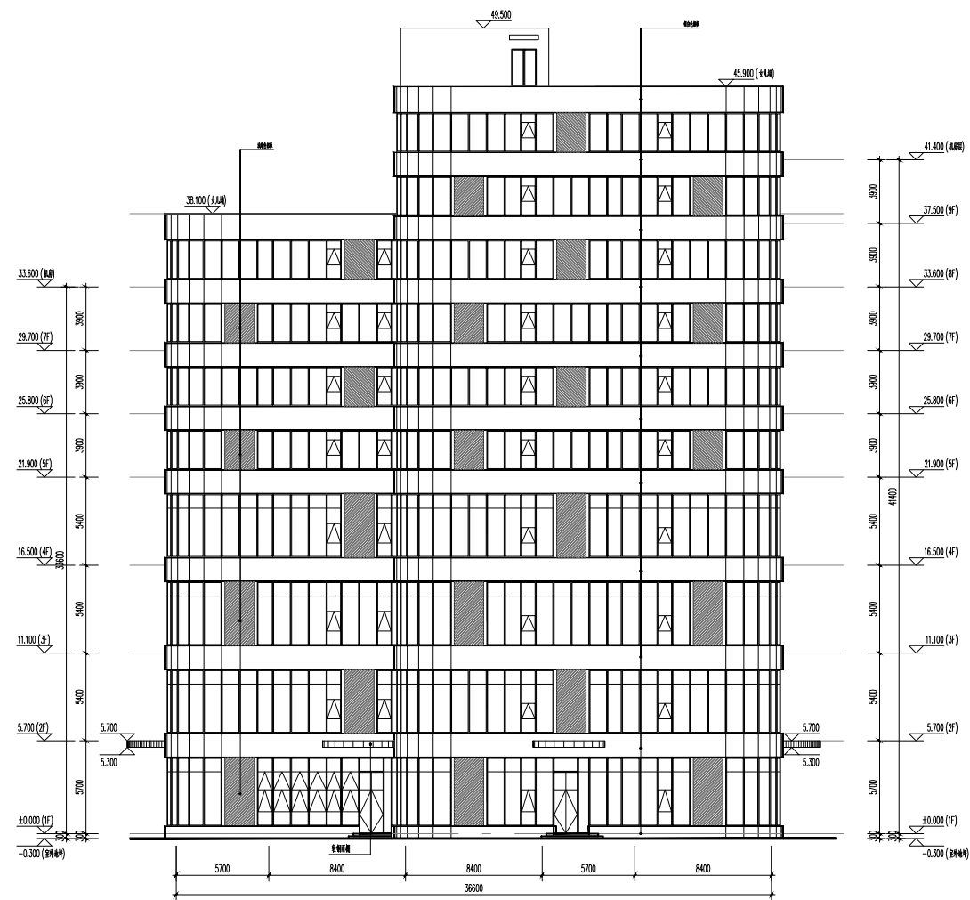
V-C 立面图 1:50
