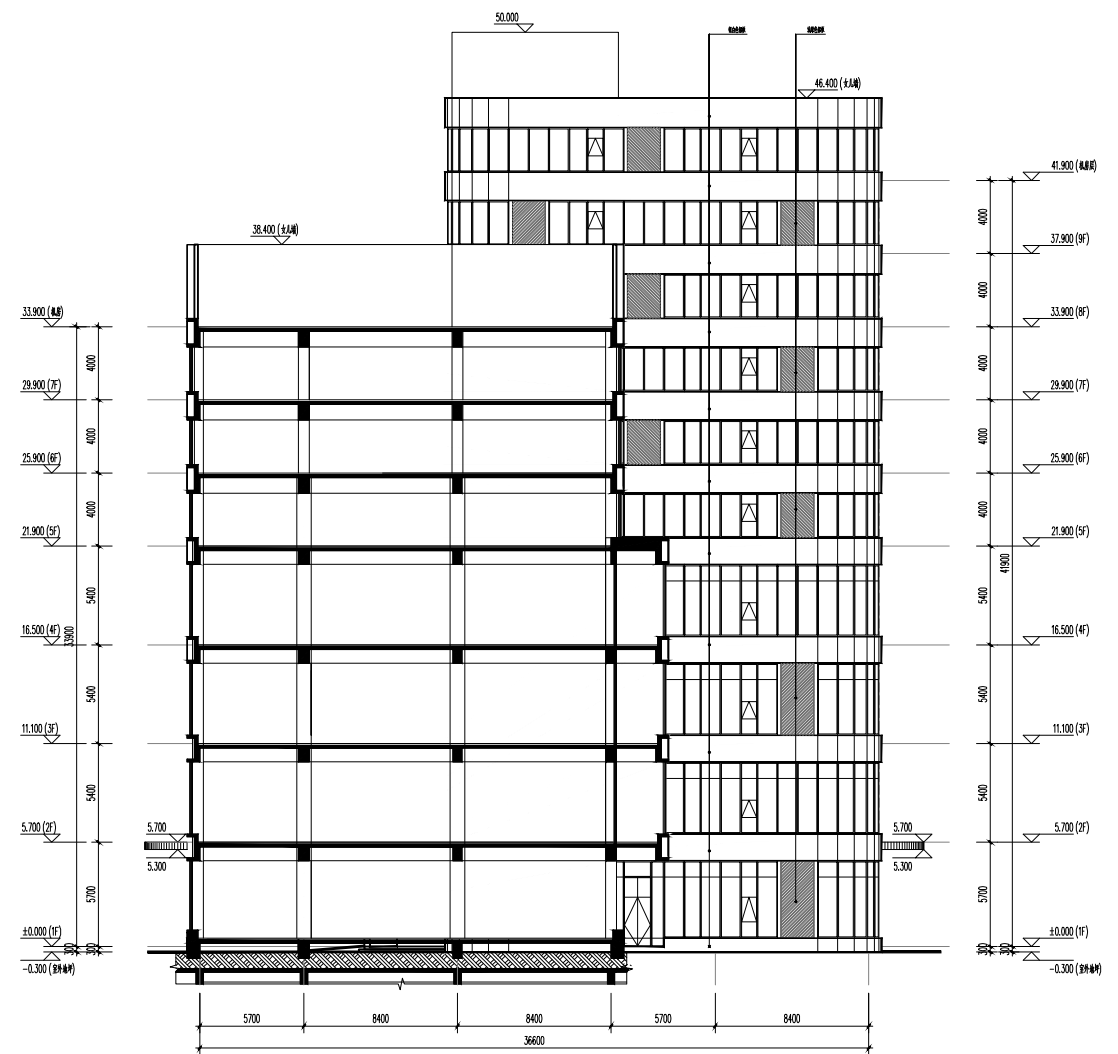
东立面图 1:50
