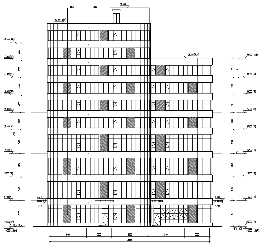
西立面图 1:50
