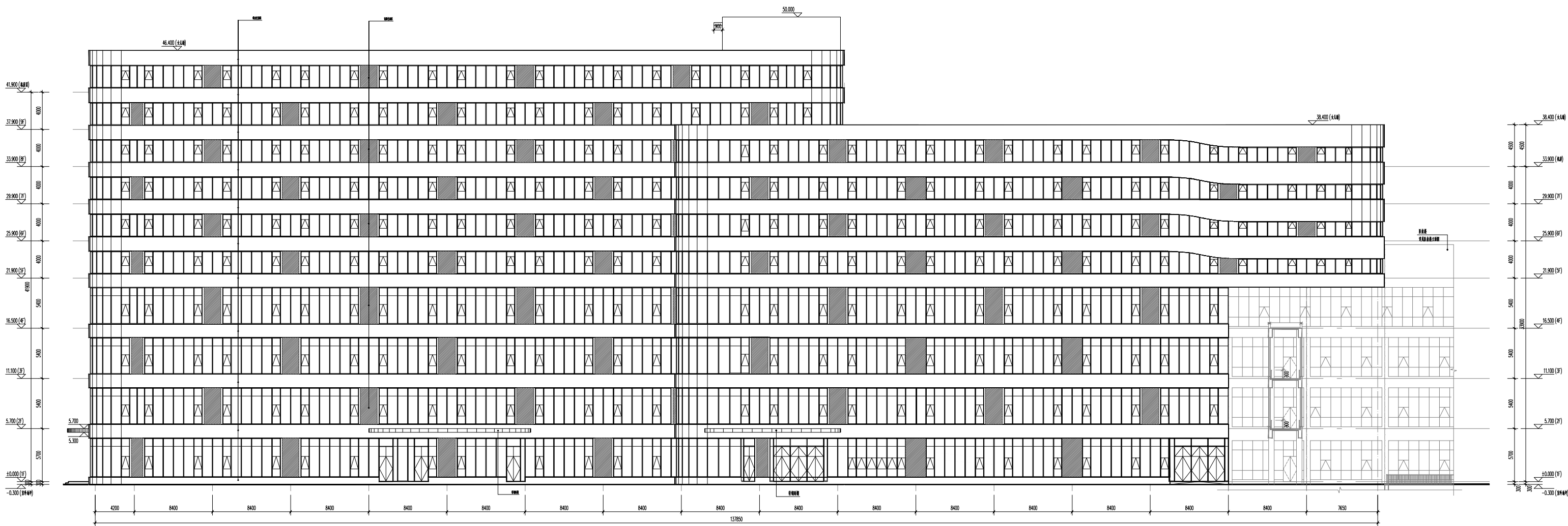
南立面图 1/50
