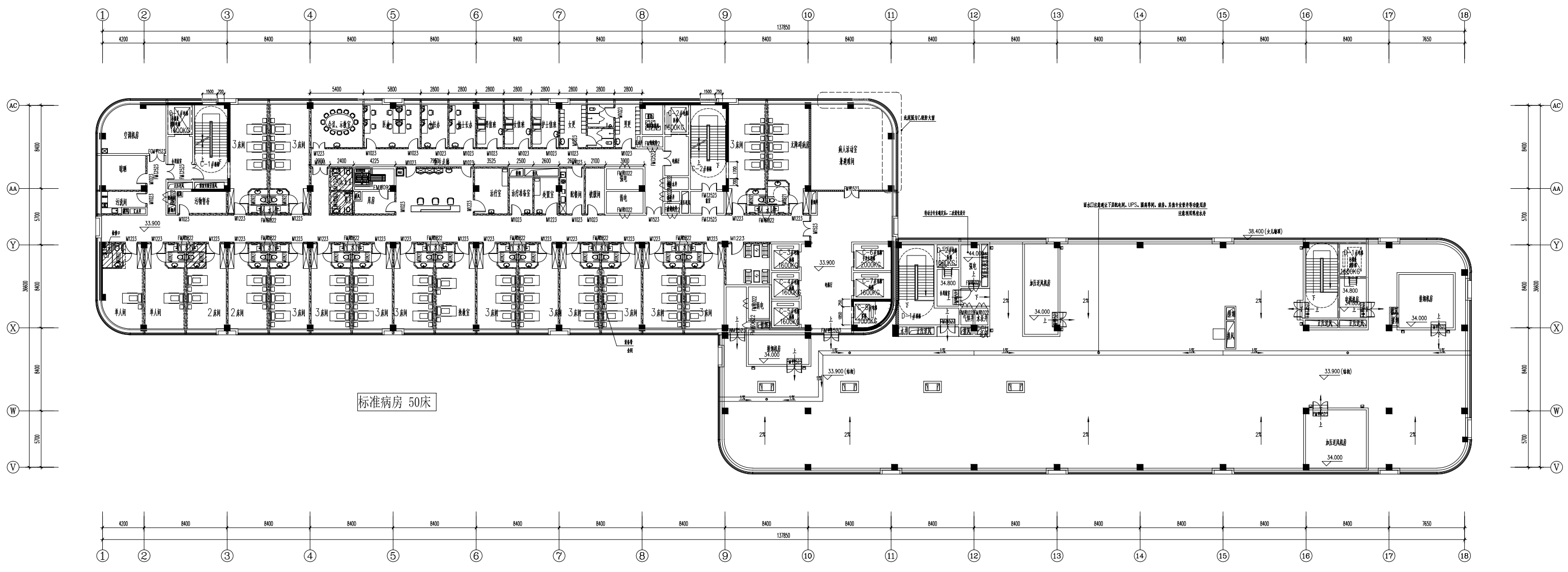
八层平面图 1:150
