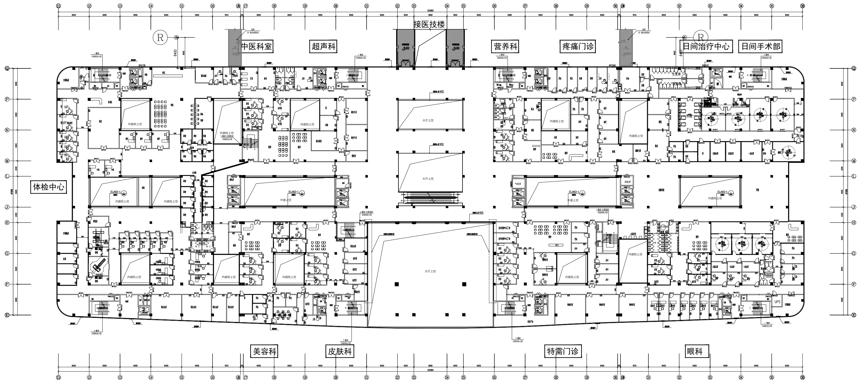
四层平面图 1:100
