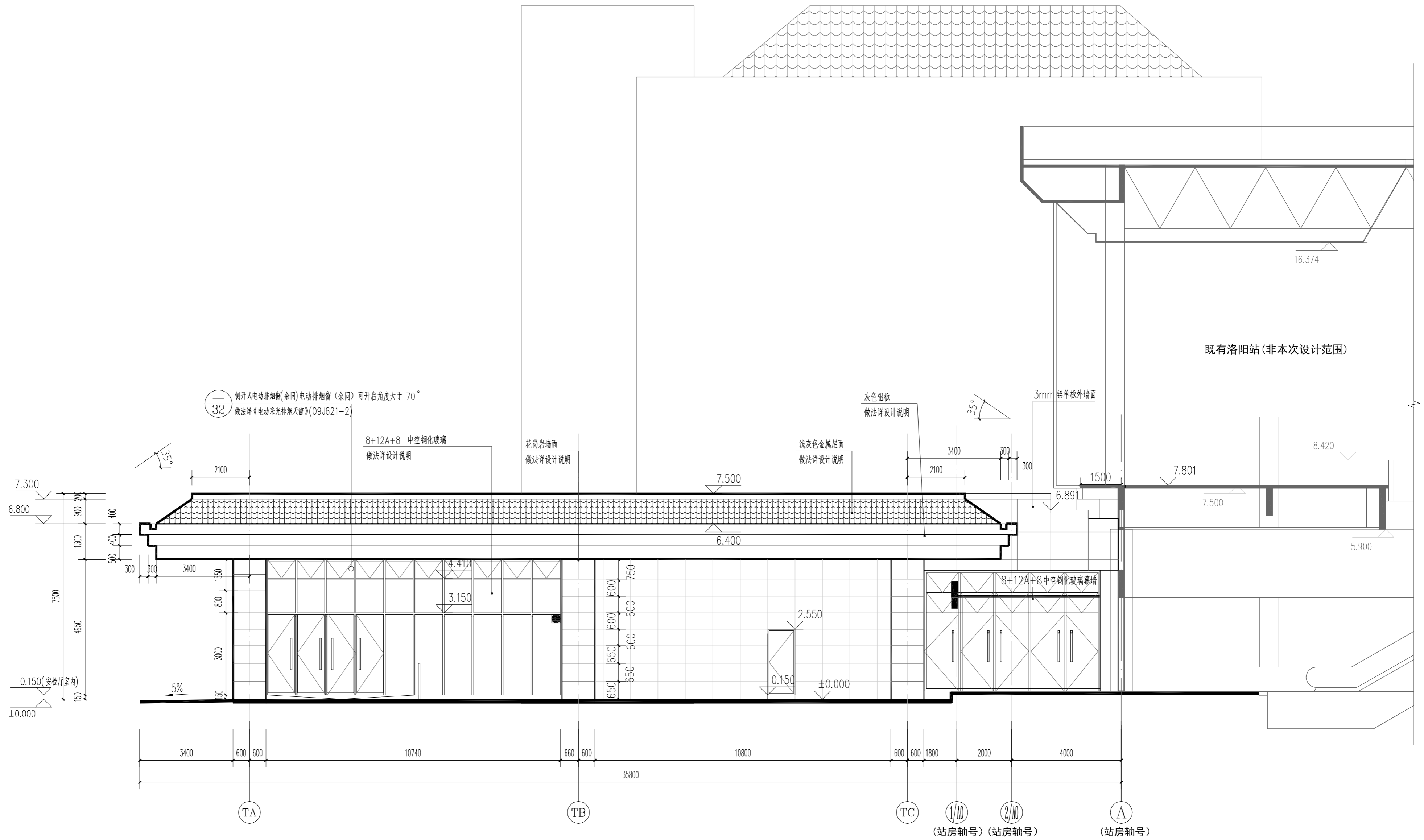
TA-TE 立面图 1:100
