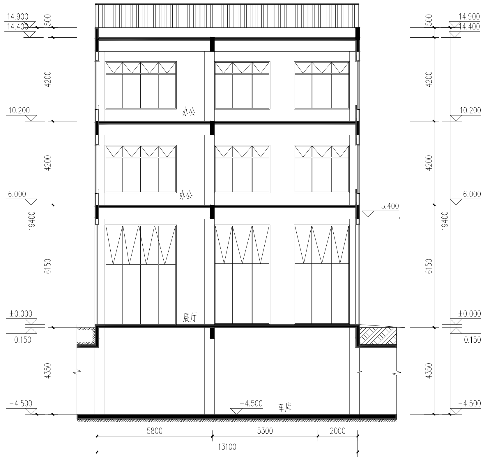
1-1剖面图
