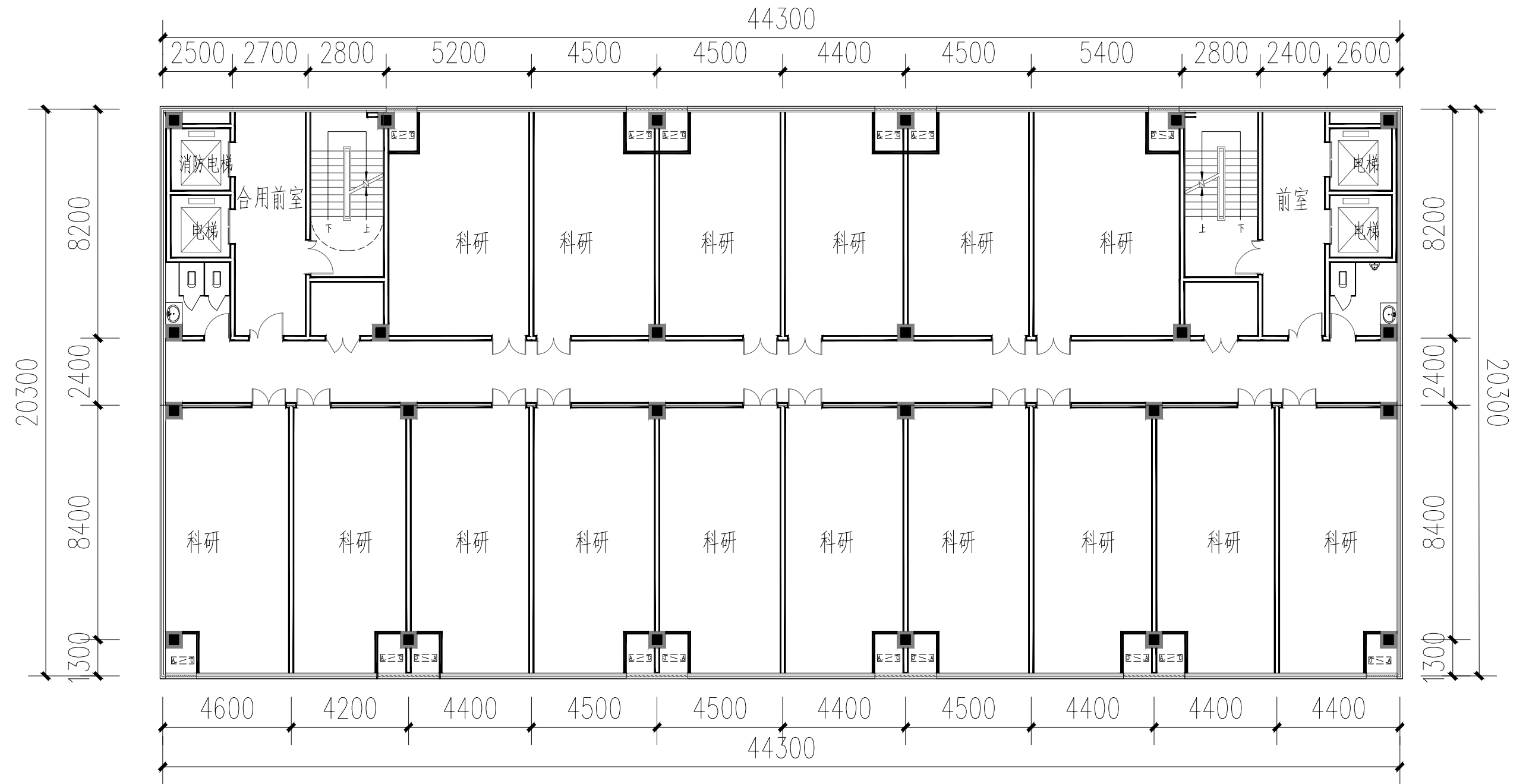
标准层平面图
