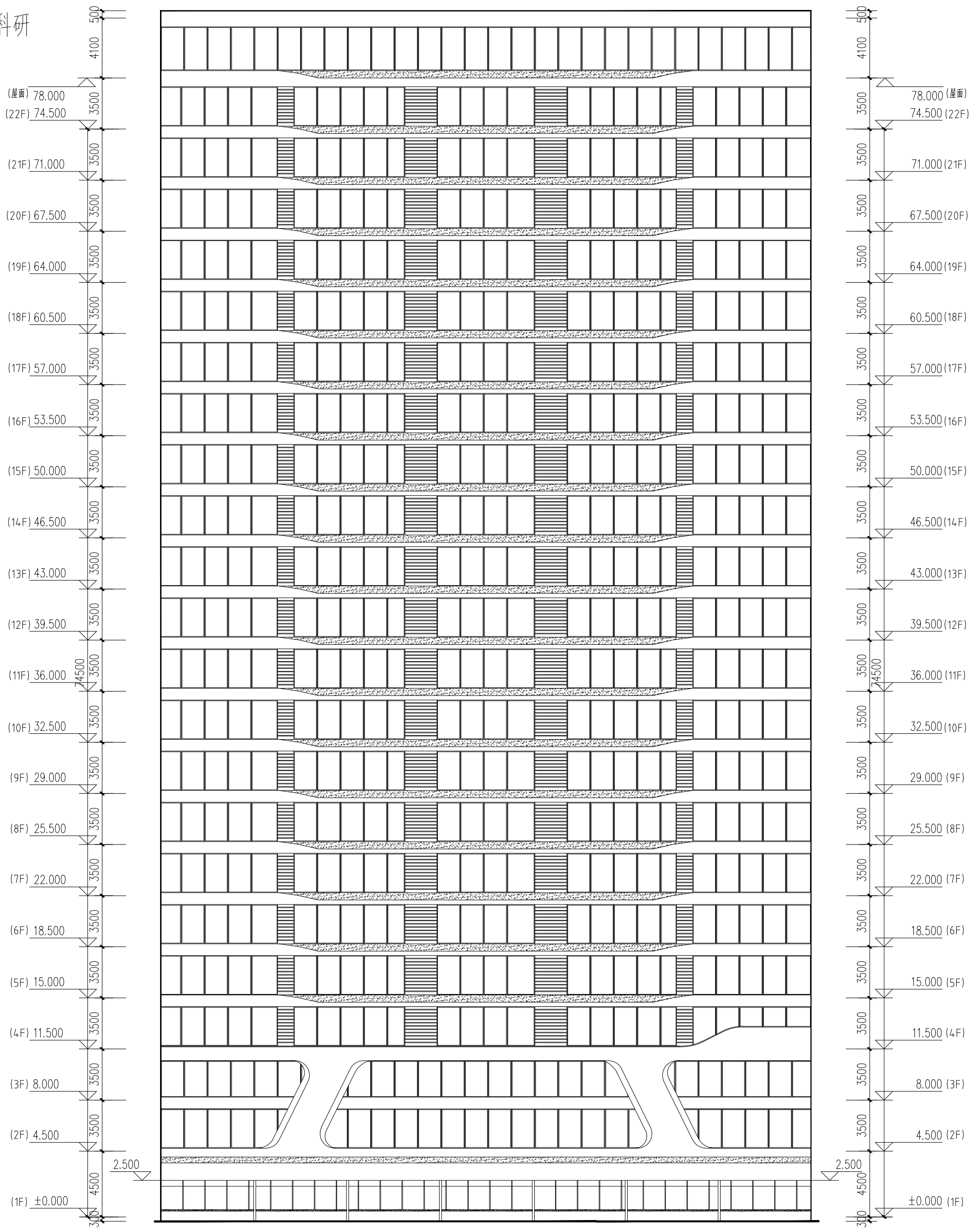
北立面图
