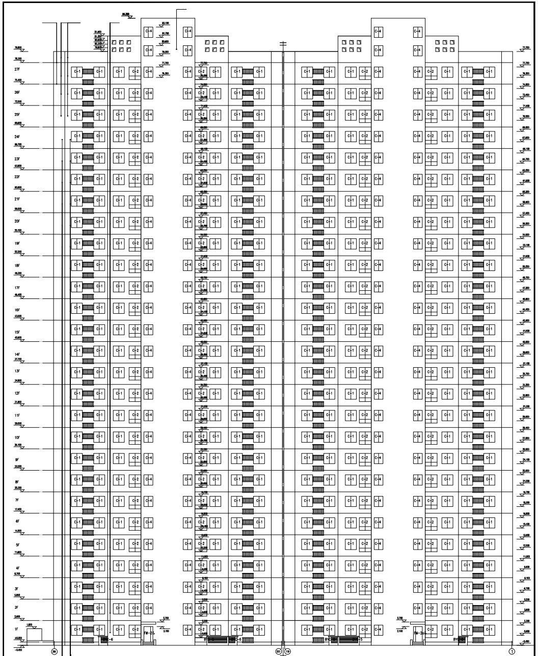
①-①平面图 1:50
