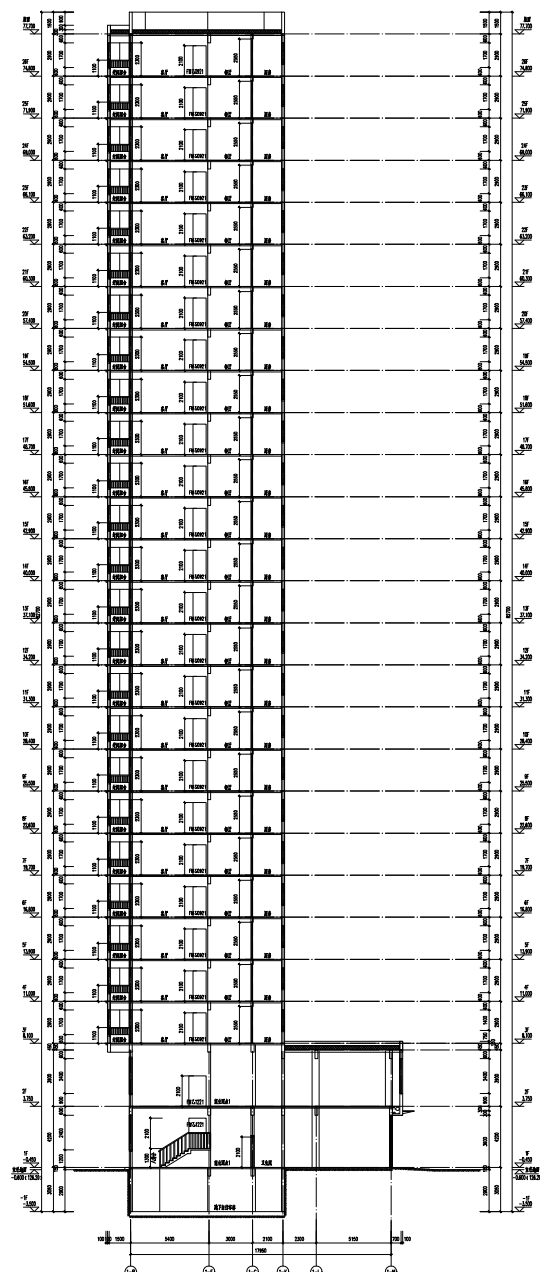
4-4剖面图 1:100
