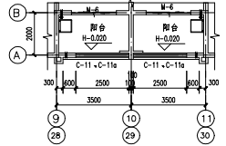
二十六二十七层局部平面图 1:100
