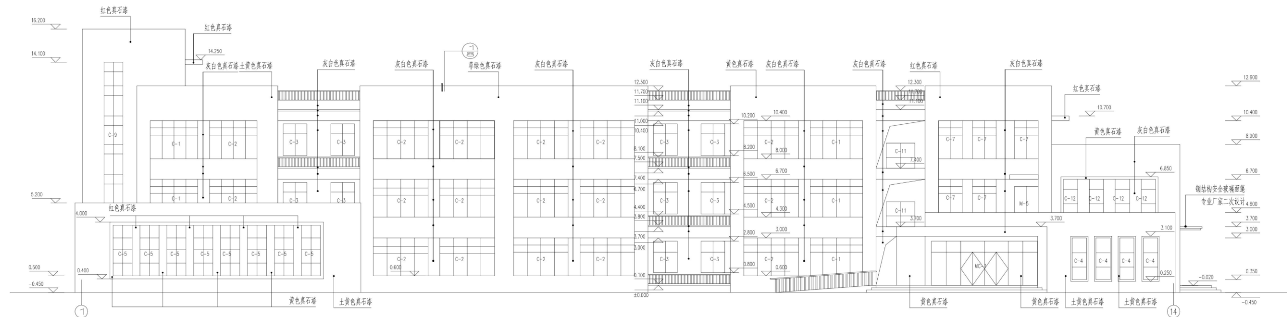
1-14 立面图 1:100
