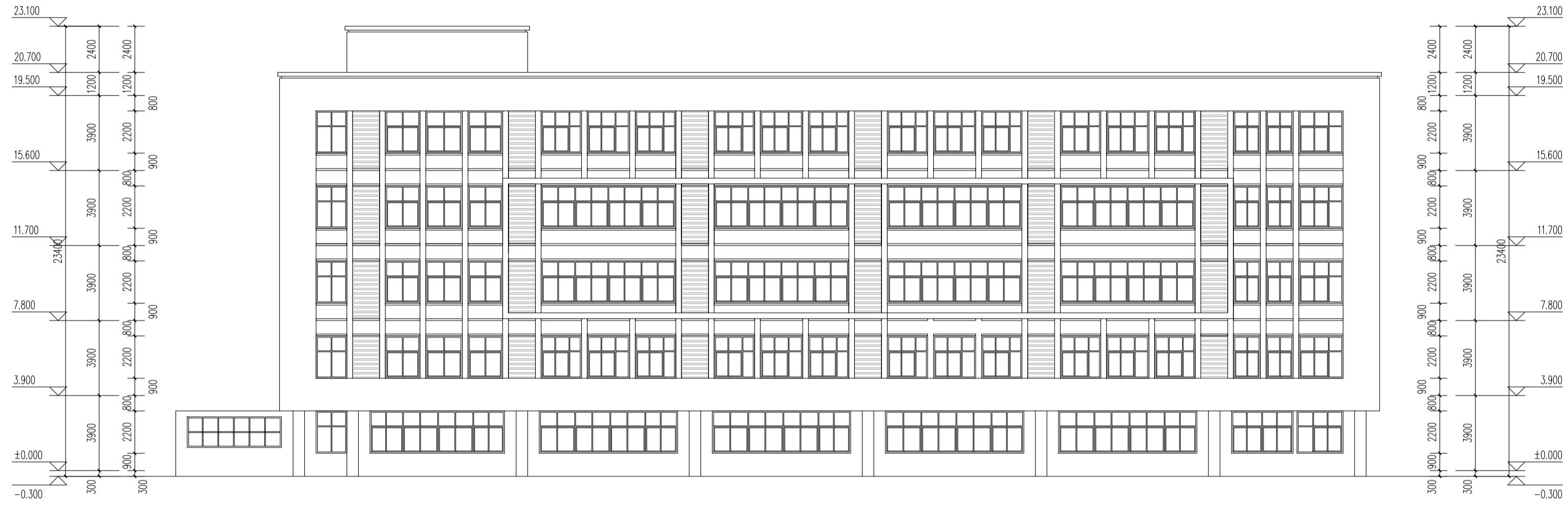
南立面图
