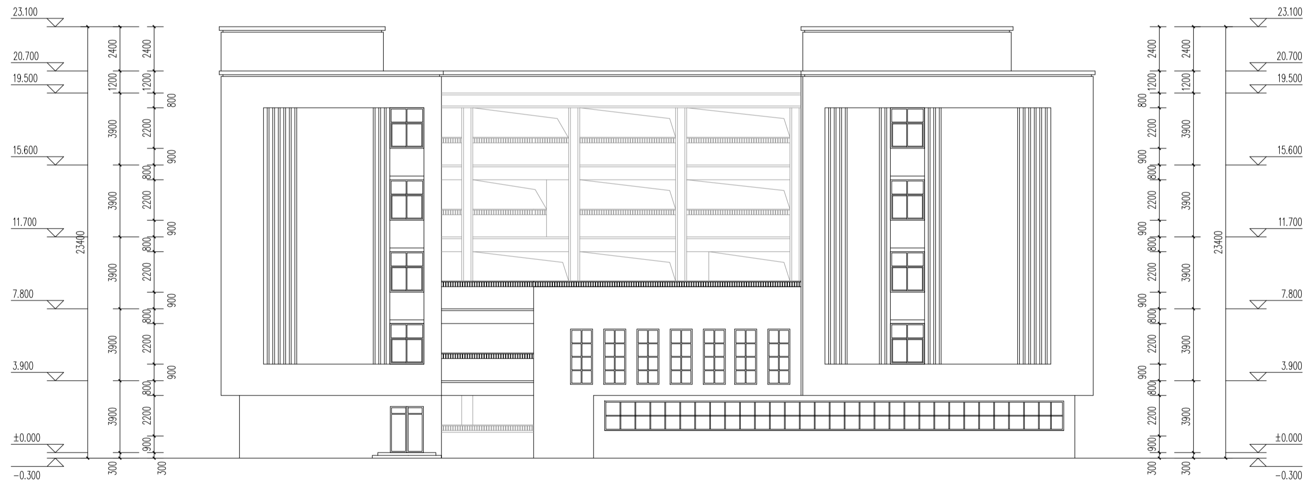
西立面图
