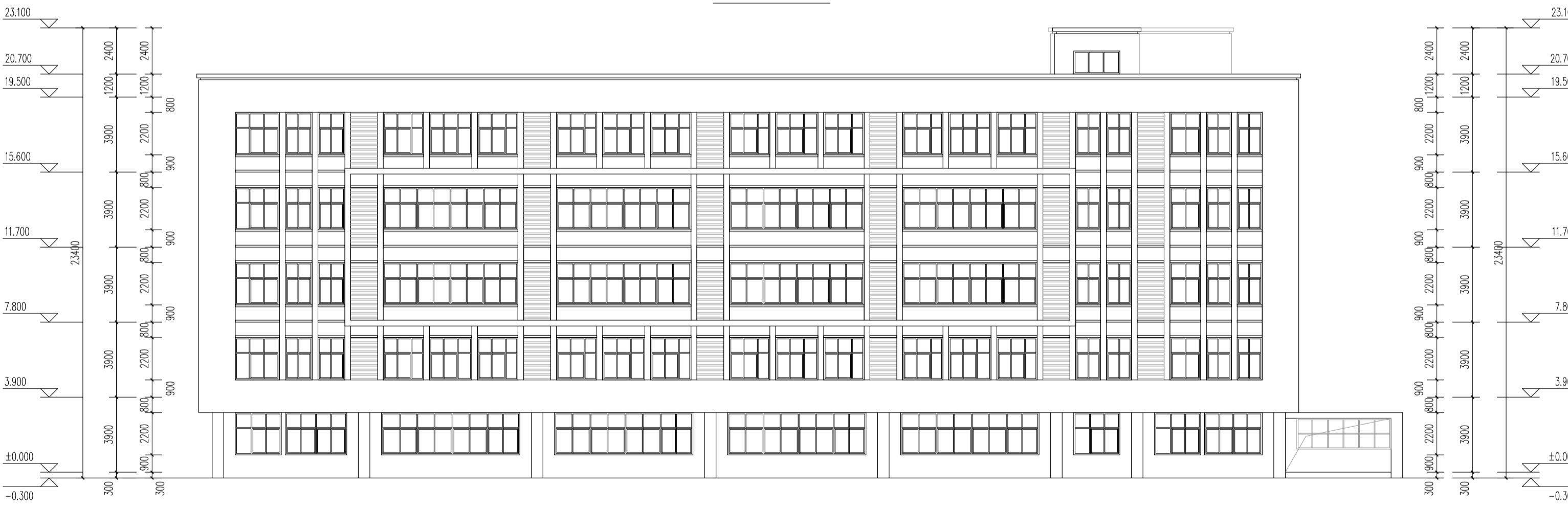
北立面图
