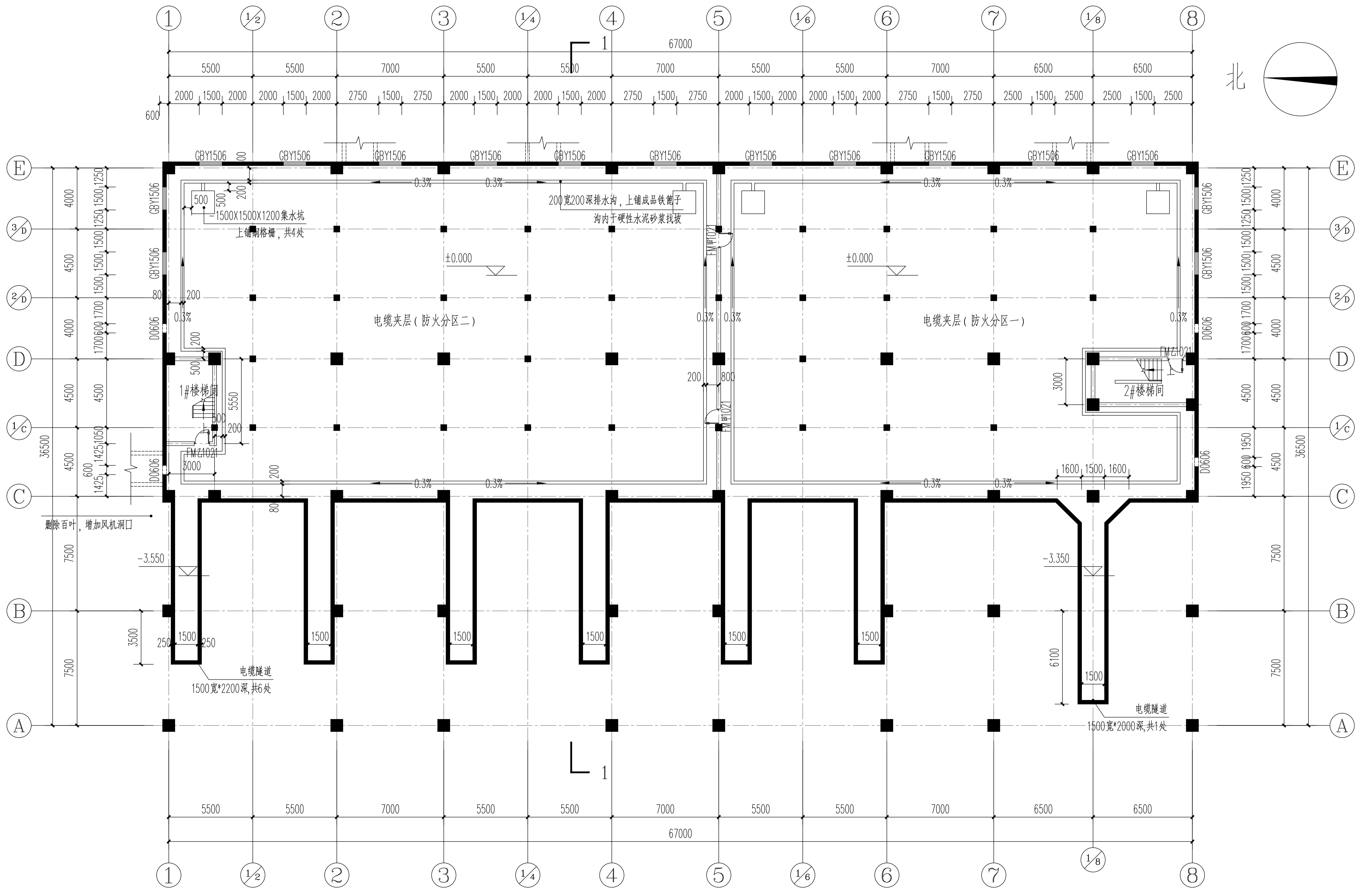
电缆夹层平面布置图 1:200 建筑面积: 1512m 2
