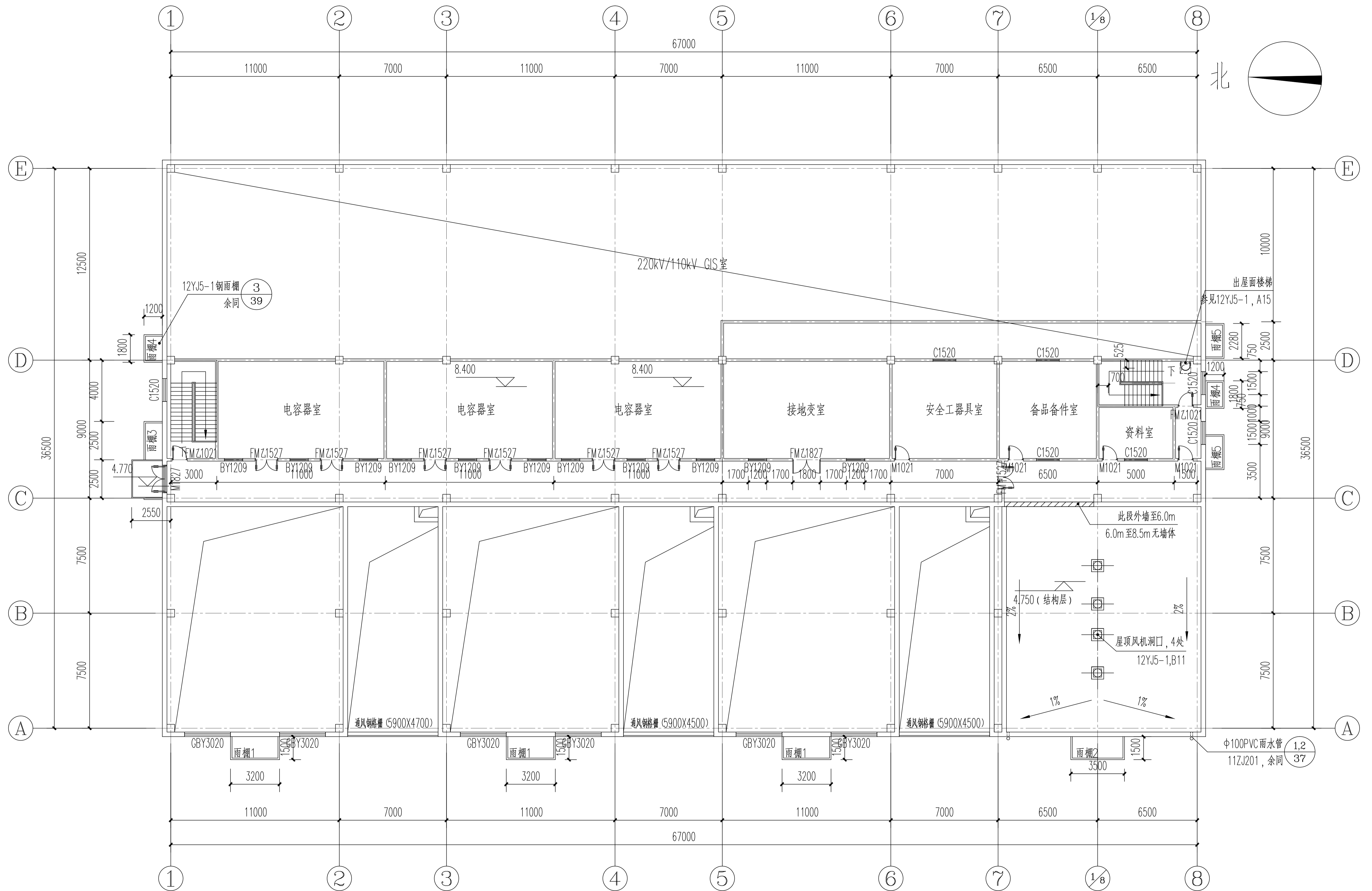
二层平面布置图 1:200 建筑面积: 686.9m 2
