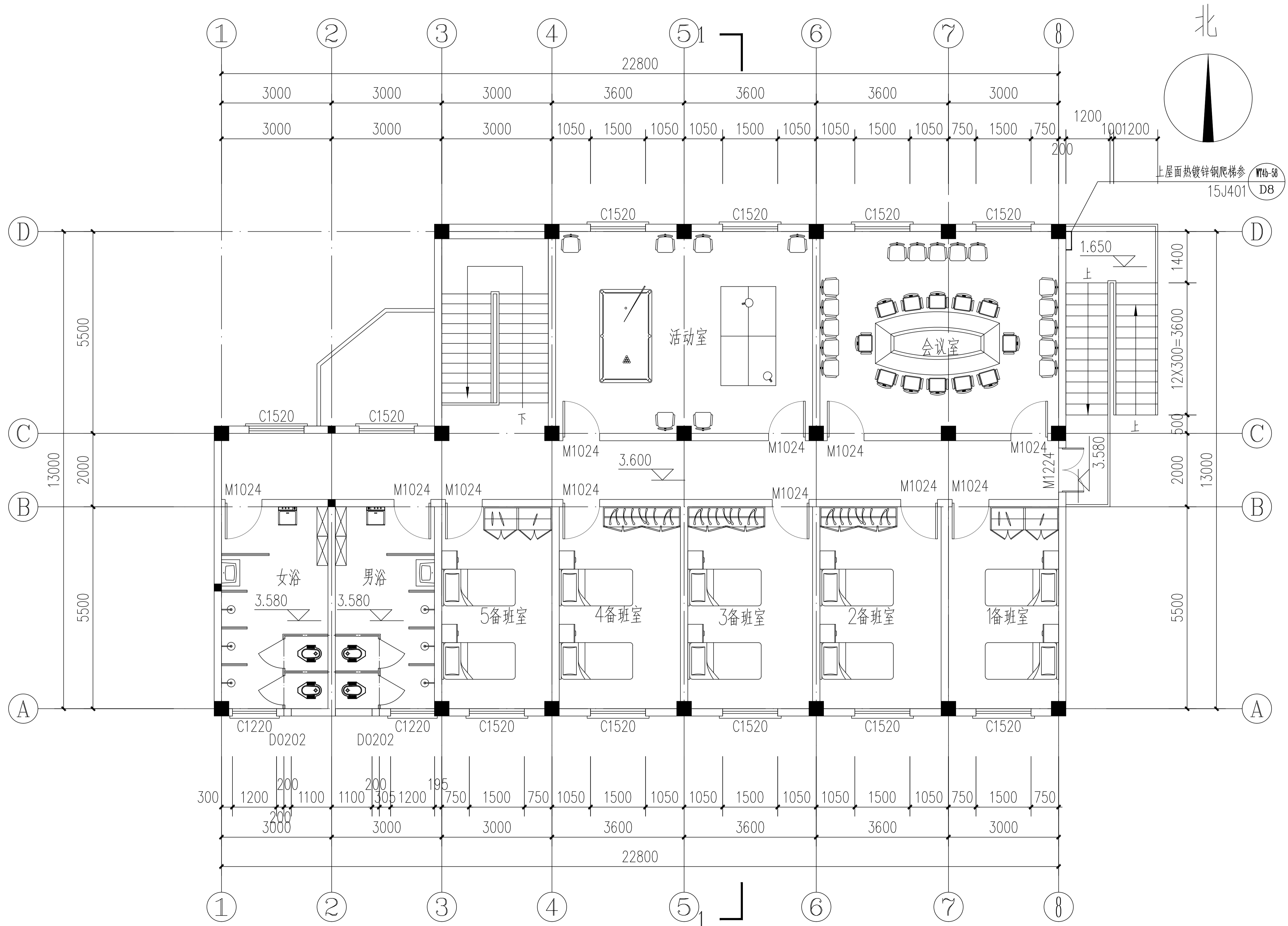
运维班用房二层平面图
