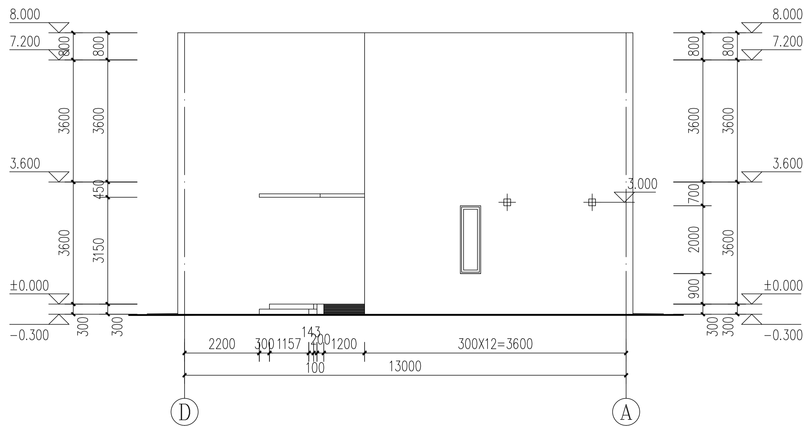
Ⓓ—Ⓐ轴立面图
