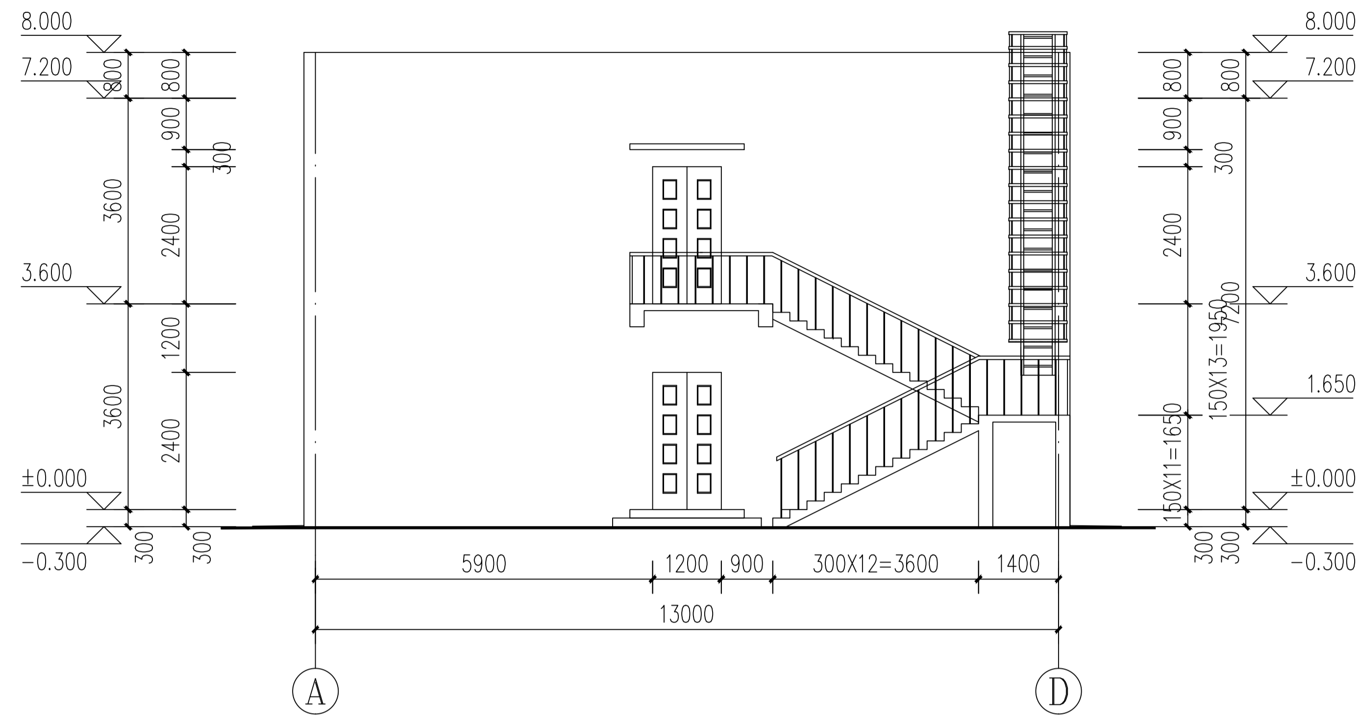
Ⓐ—Ⓓ轴立面图
