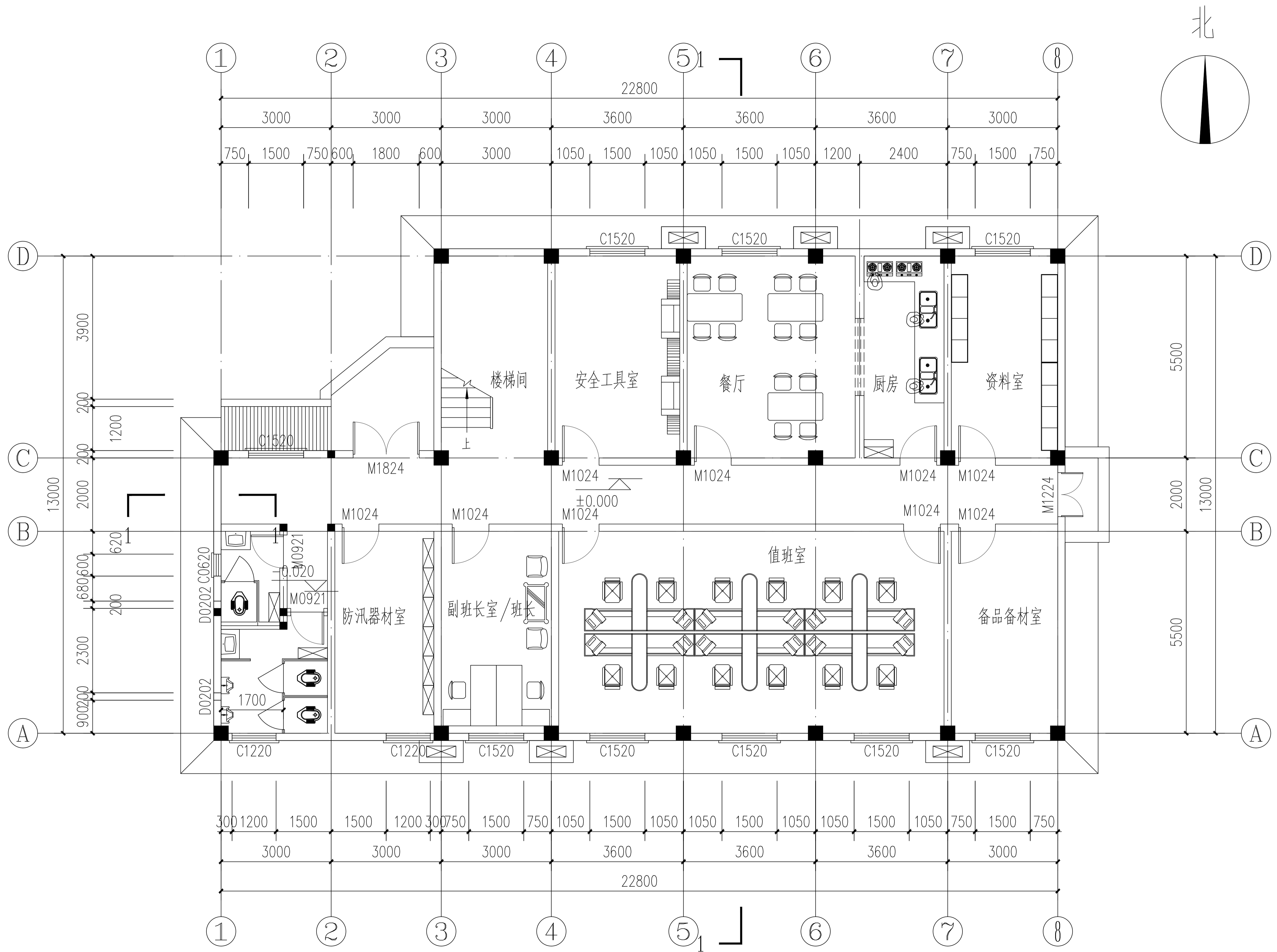
运维班用房一层平面图
