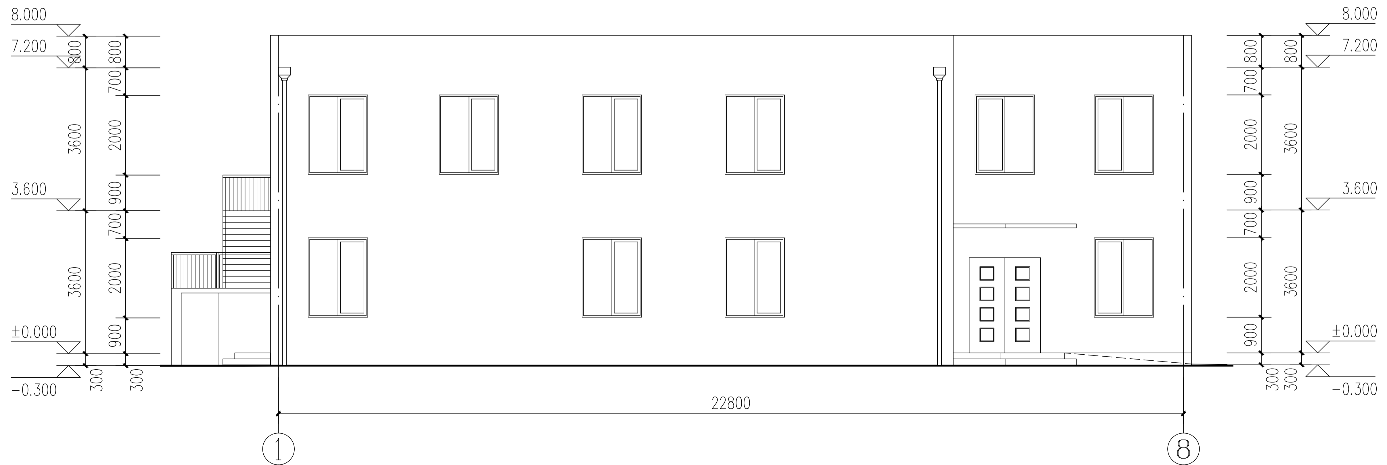
⑧—①轴立面图
