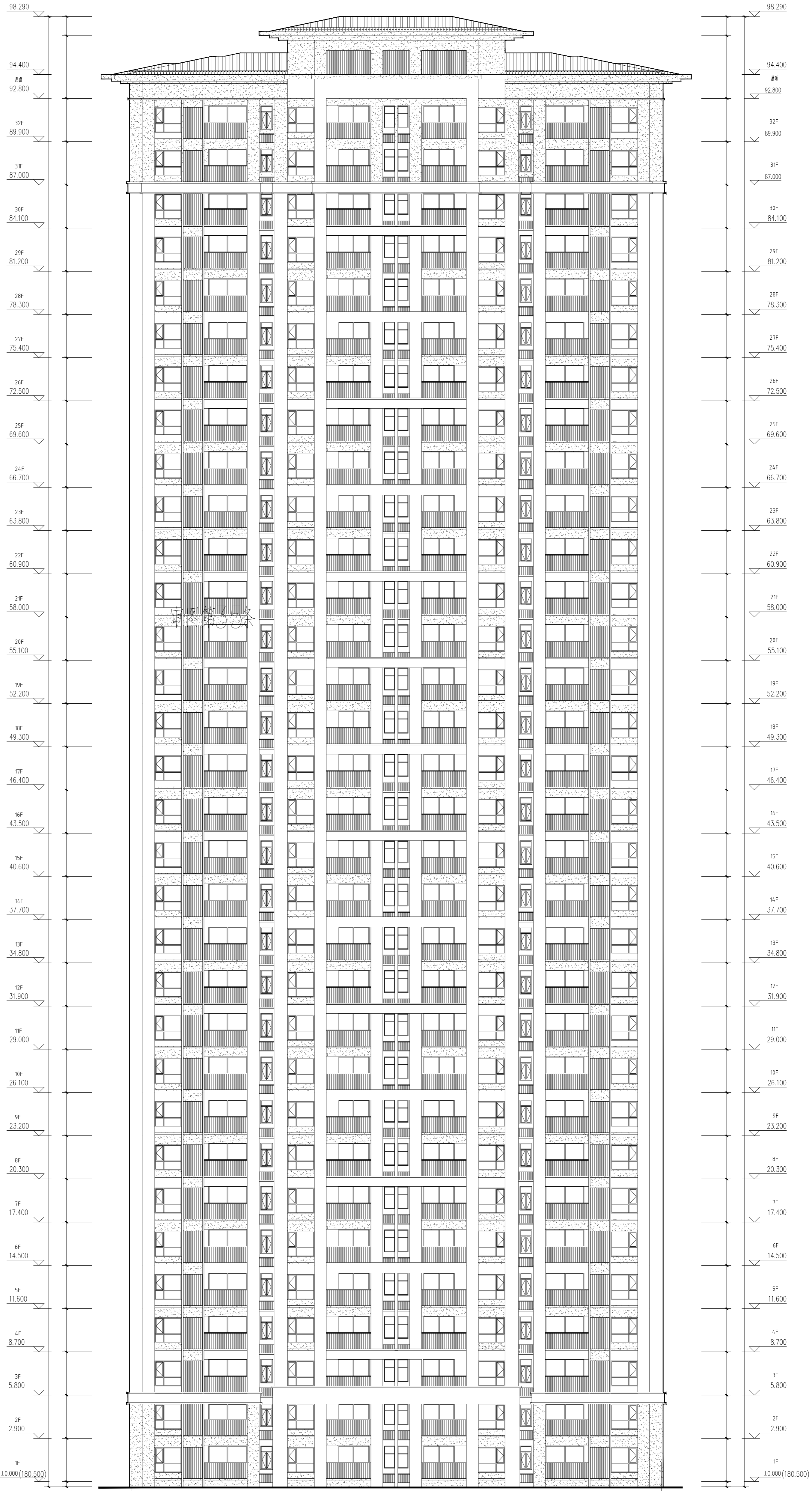
7-1 7-24 轴立面图 1:120
