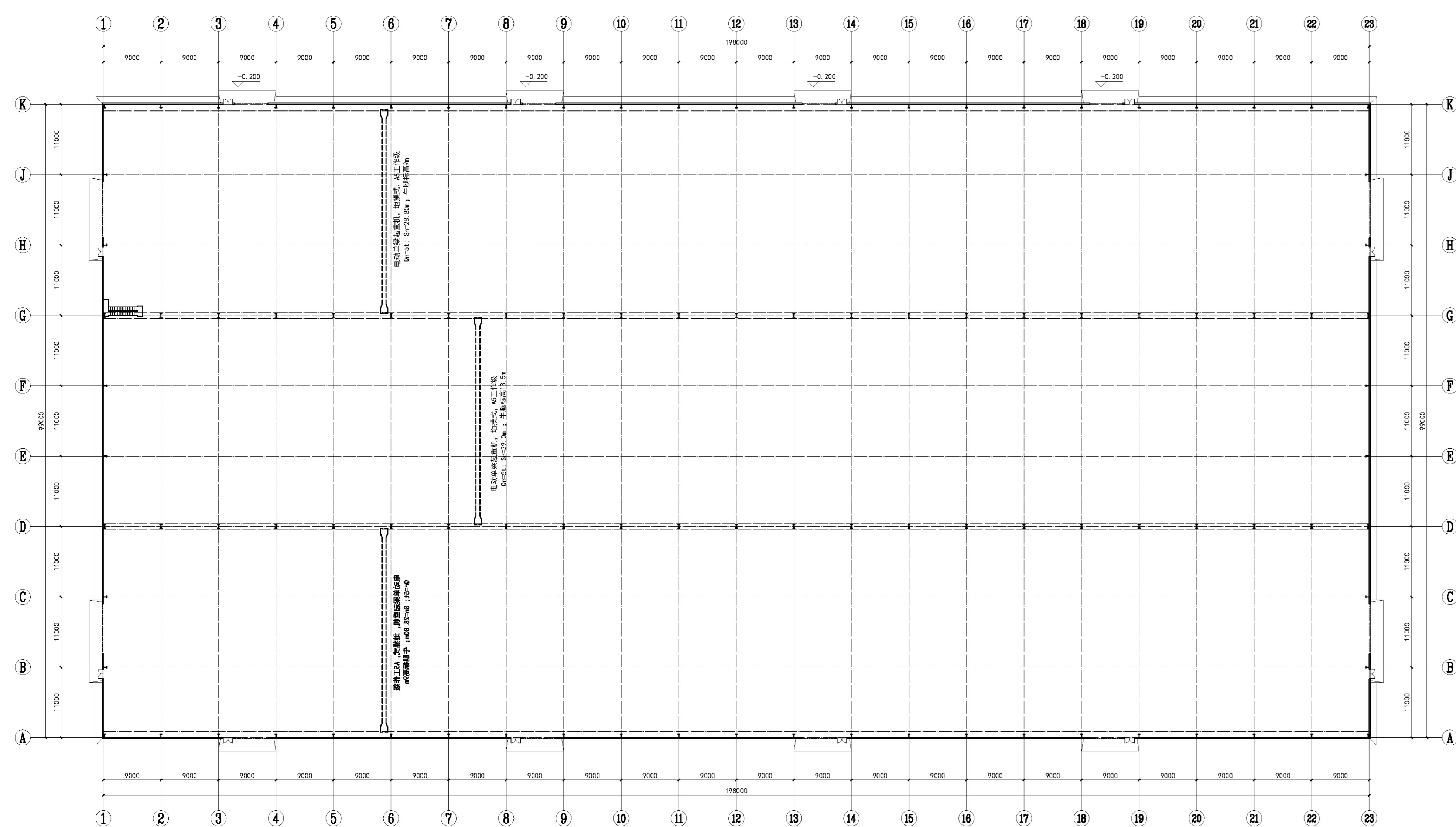
仓库一层平面图
