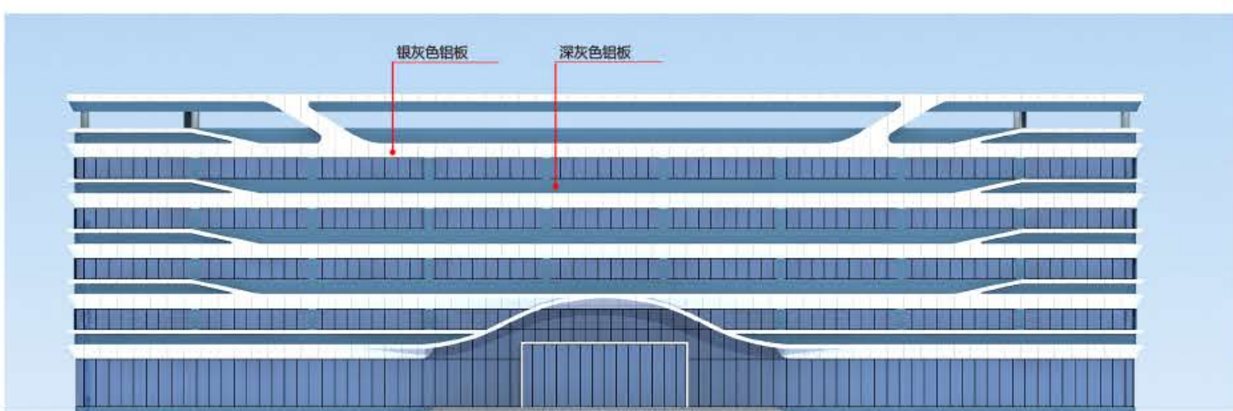
研发中心正立面图
