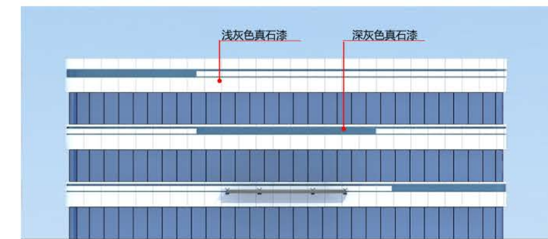
运营楼立面图
