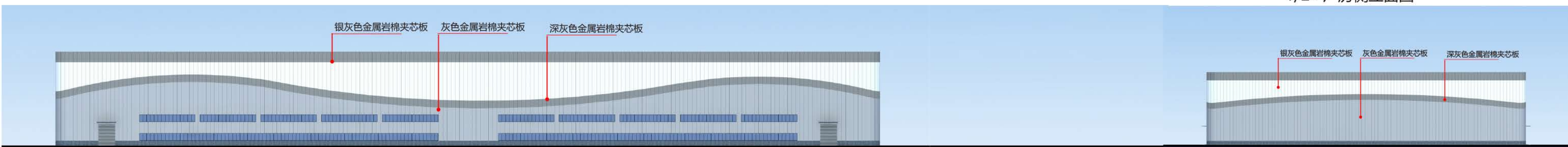
仓库正立面图
