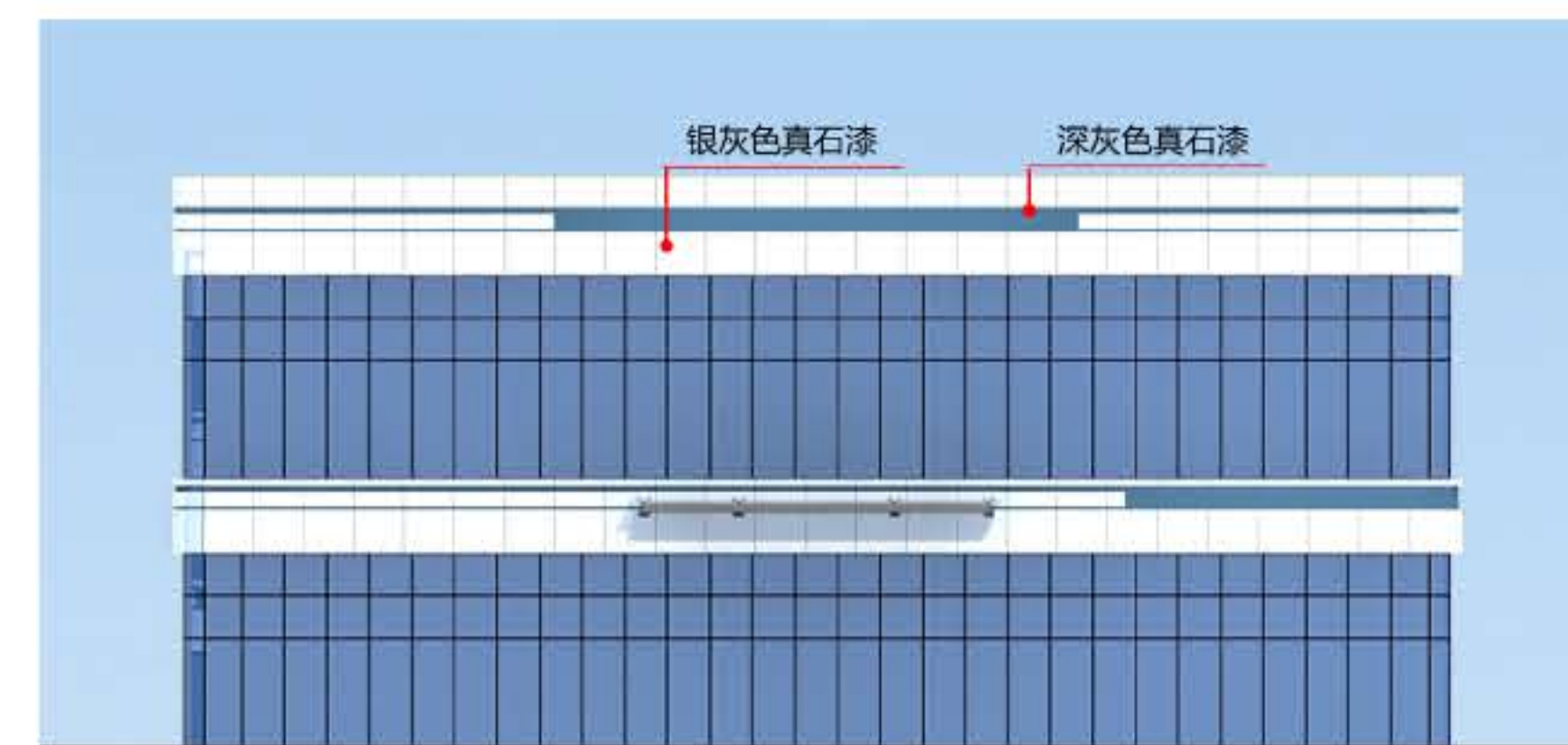
综合站房（开闭所、水泵房、制氮站）立面图
