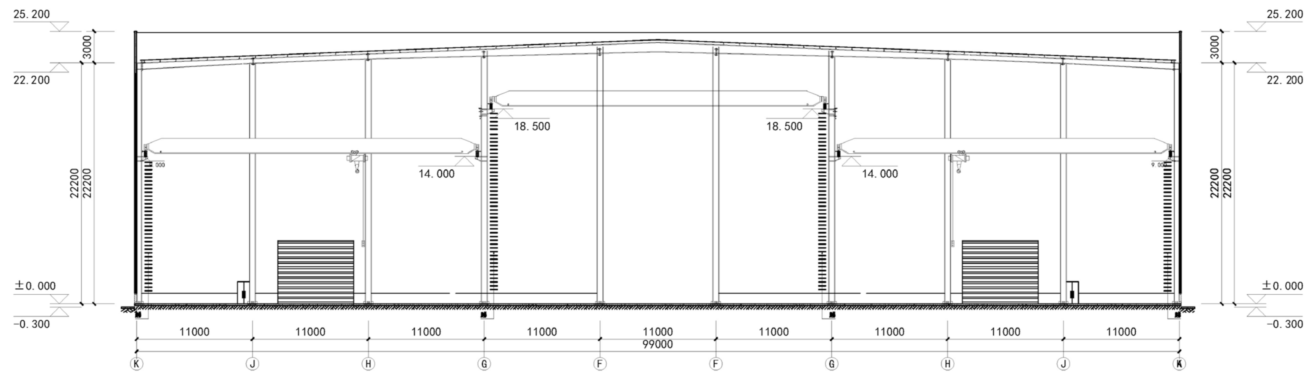
仓库剖面图
