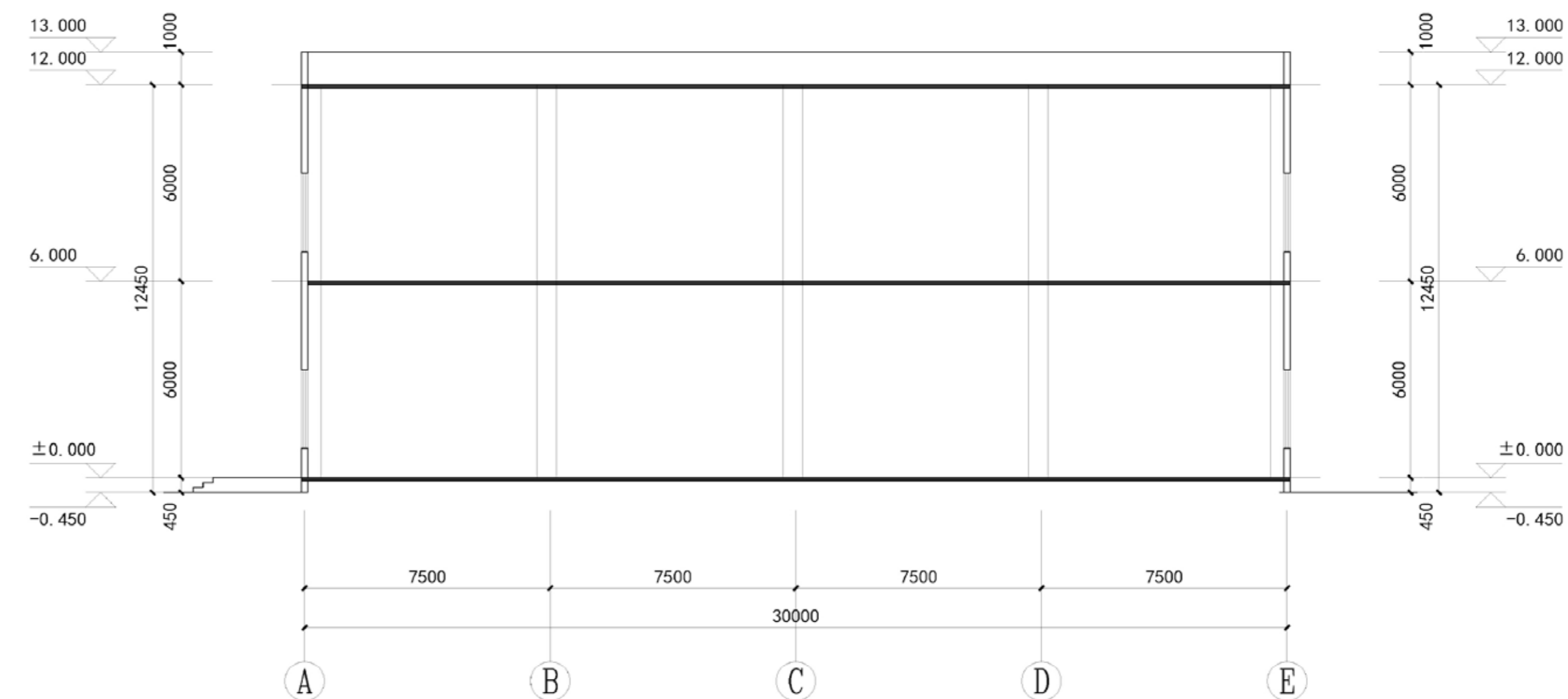
综合站房 (开闭所、水泵房、制氮站) 剖面图
