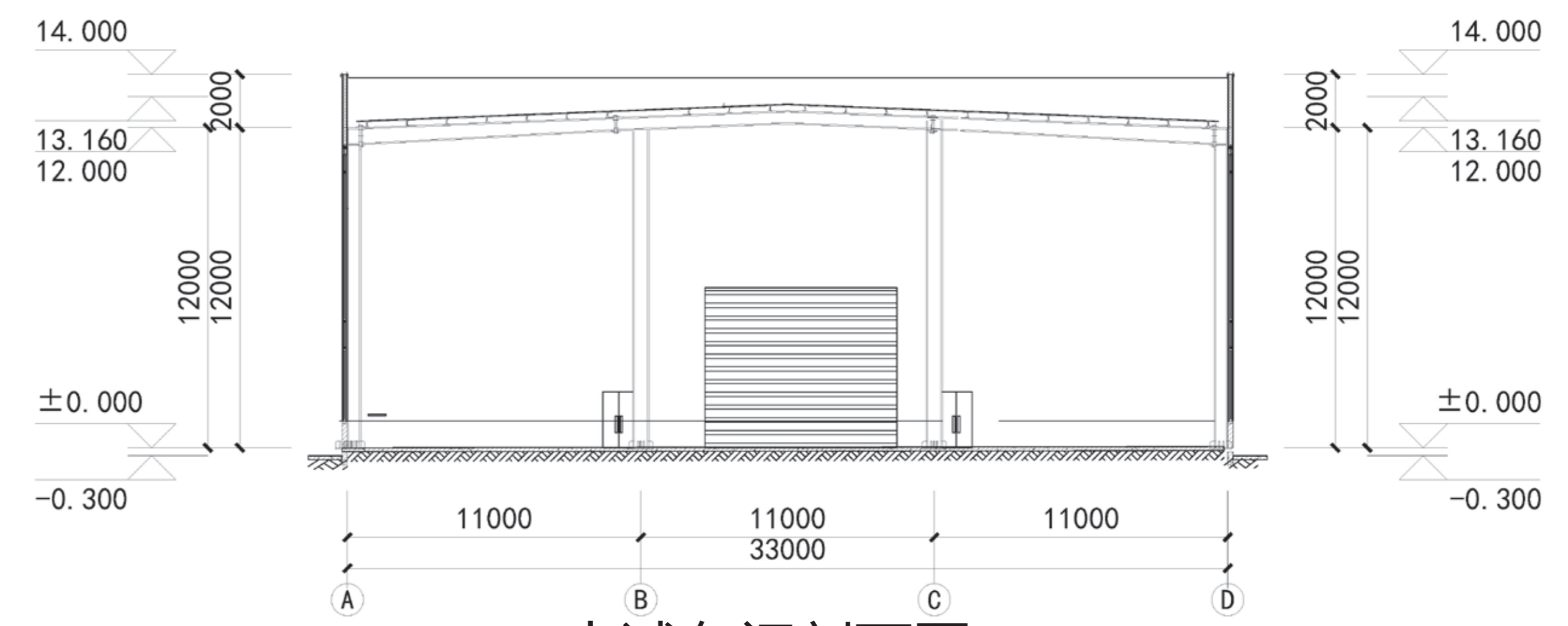
中试车间剖面图
