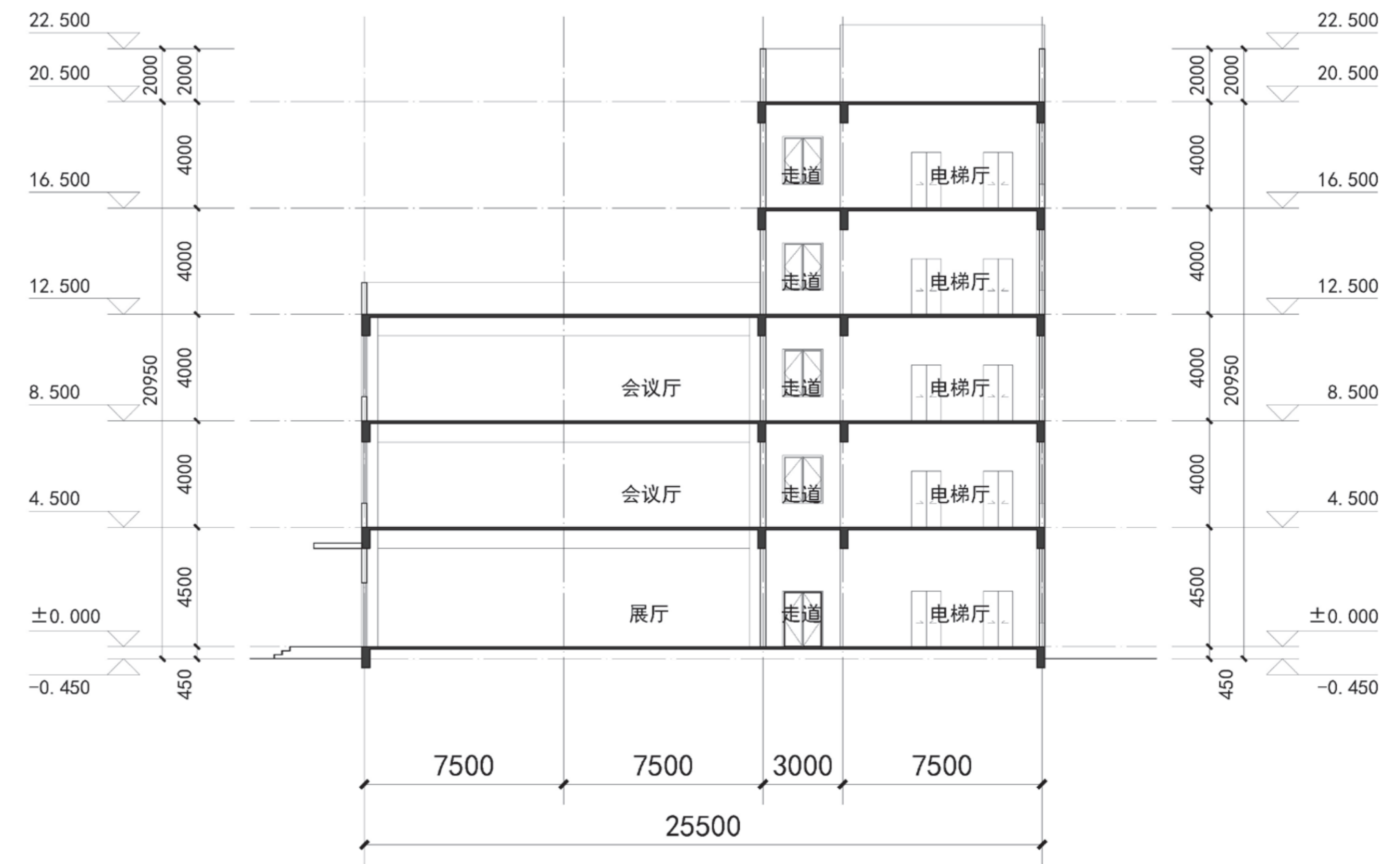
研发中心剖面图
