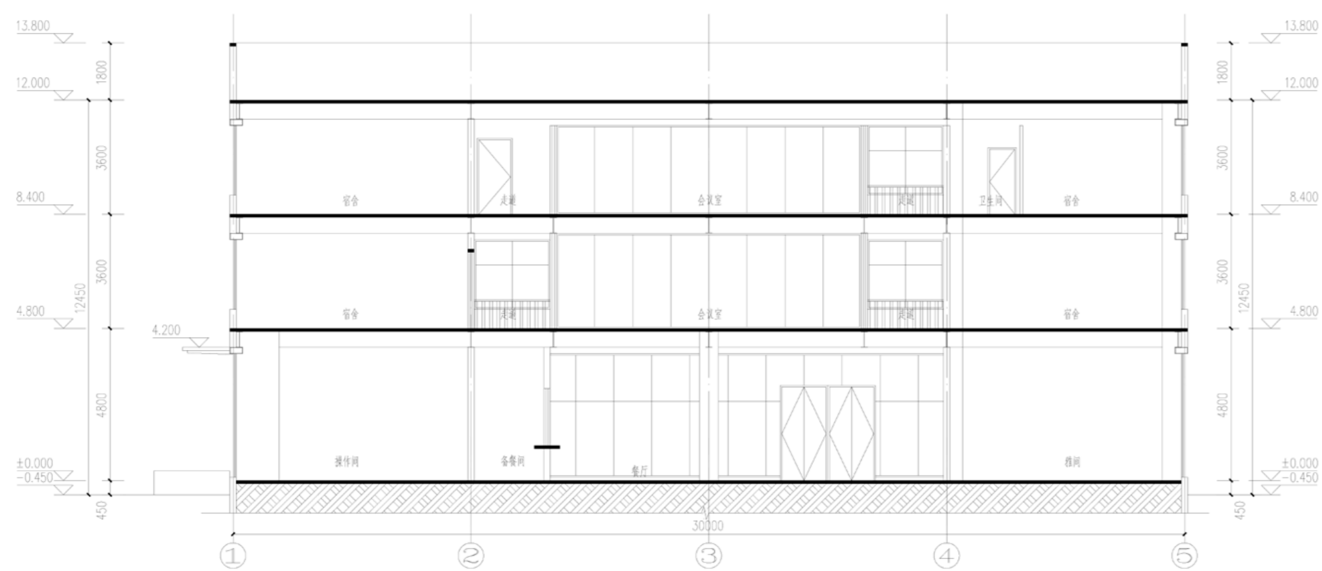
运营楼剖面图
