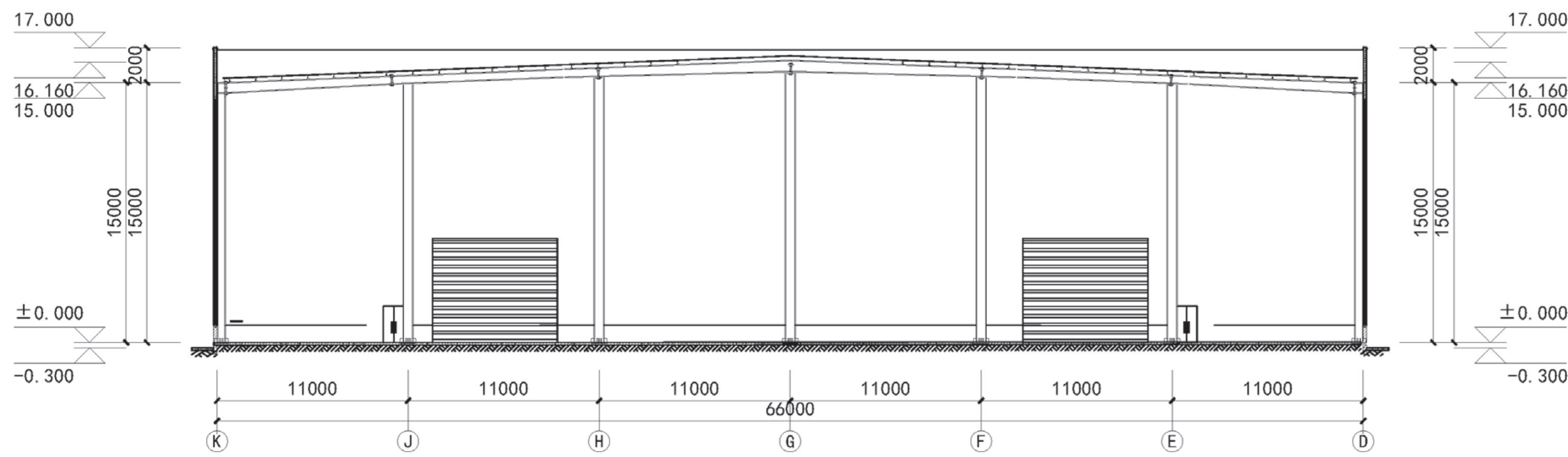
1/2# 厂房剖面图
