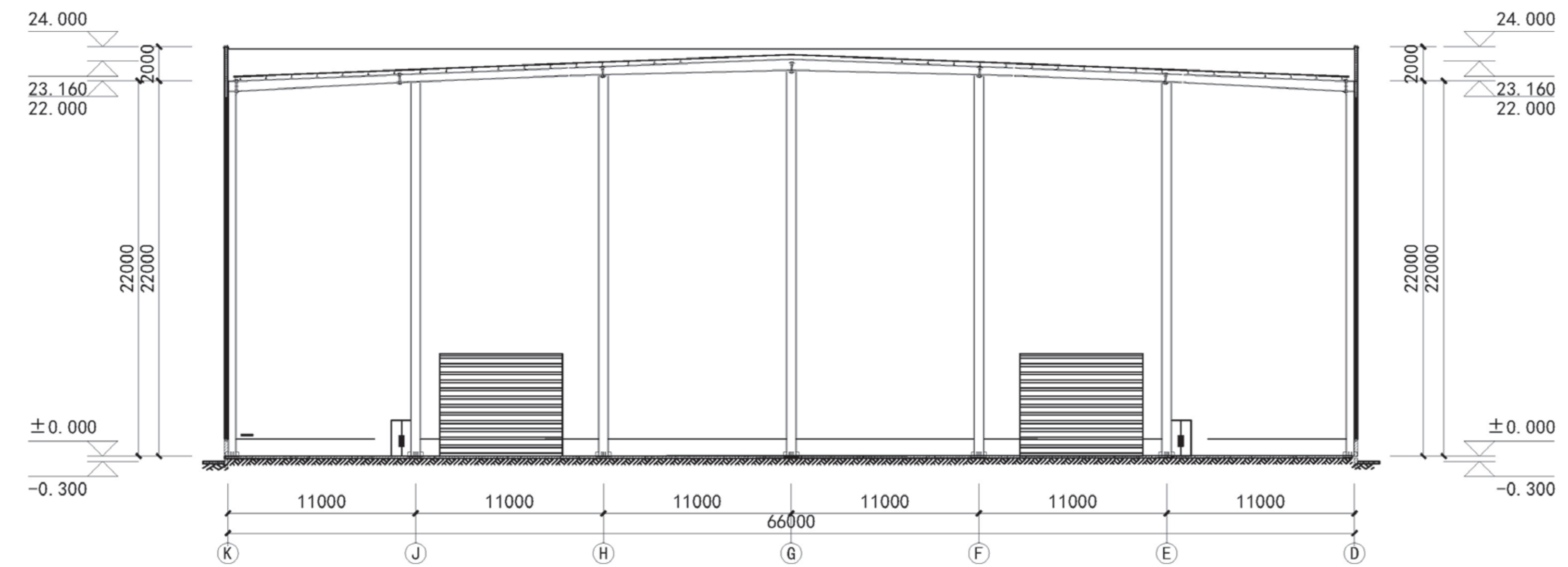
成品车间剖面图
