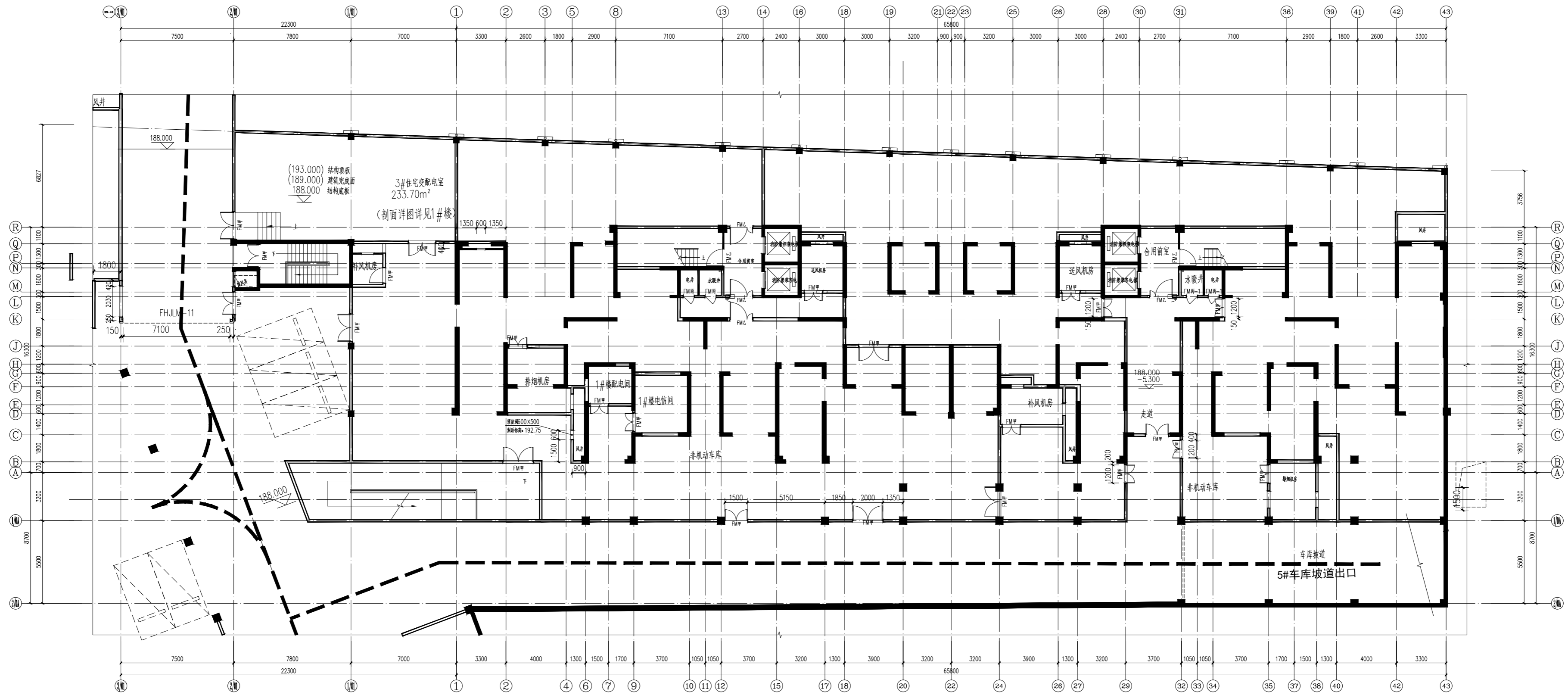
地下一层平面图 1:100
