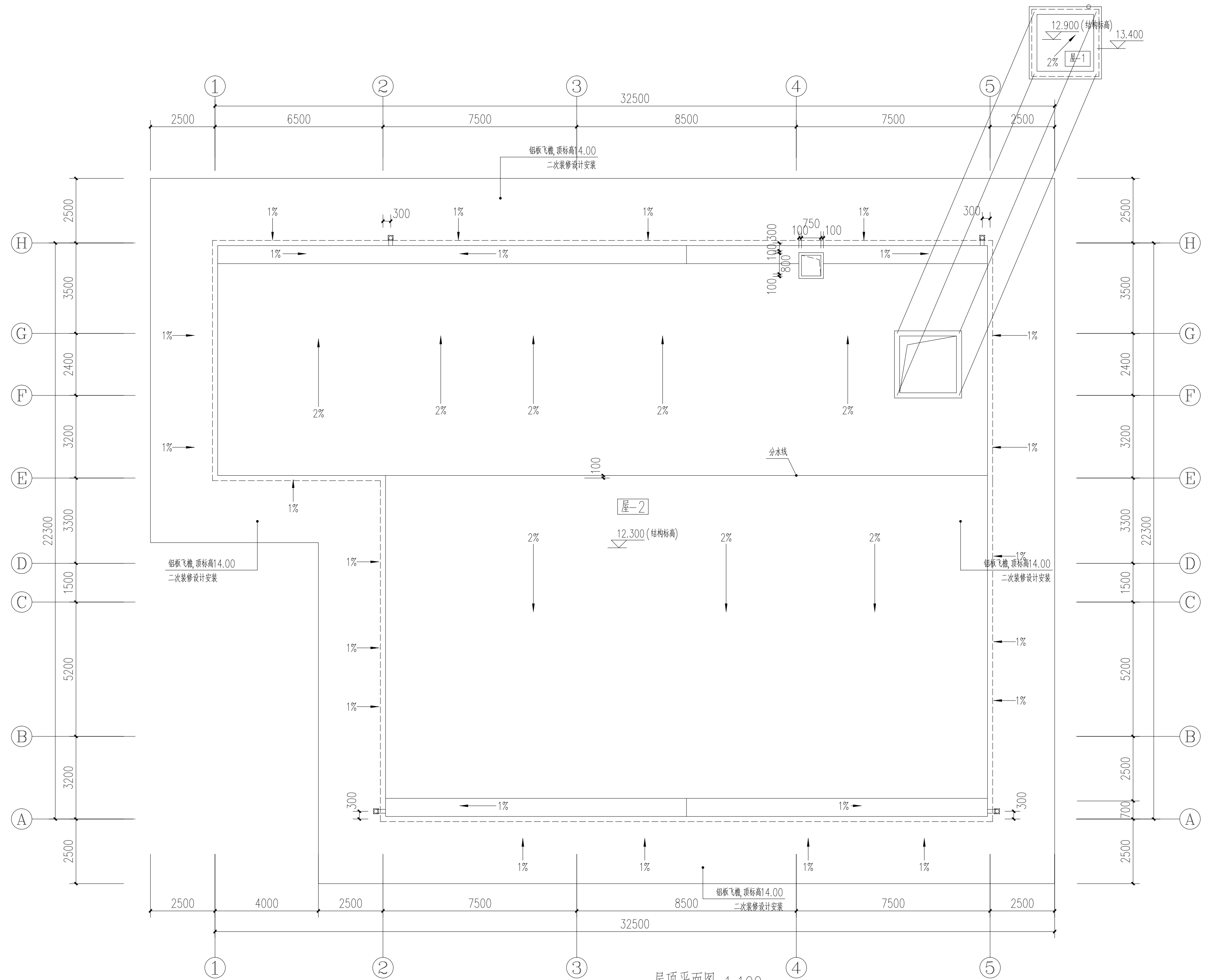
屋顶平面图 1:100
