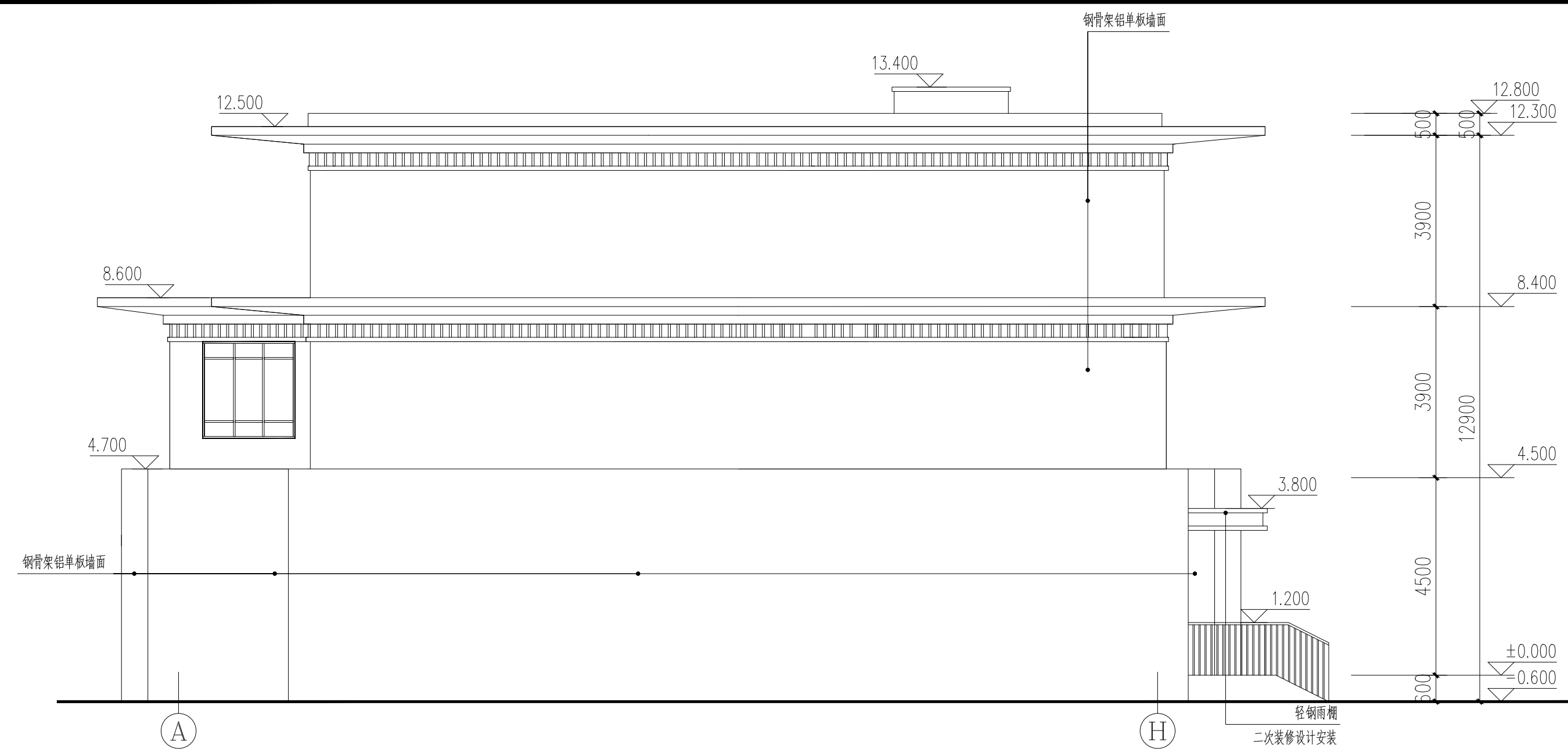
(A)-(H)立面图 1:100
