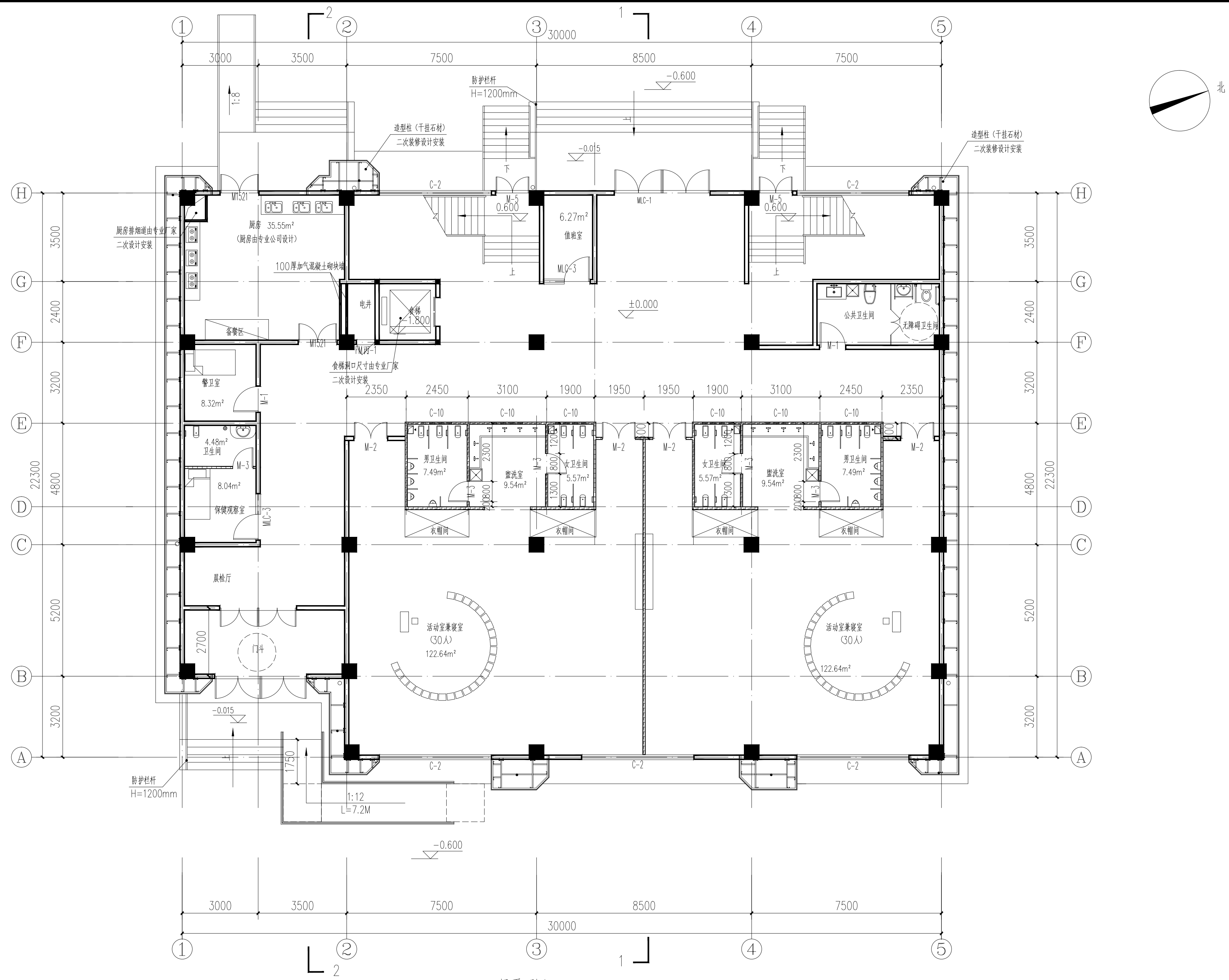
一层平面图 1:100
