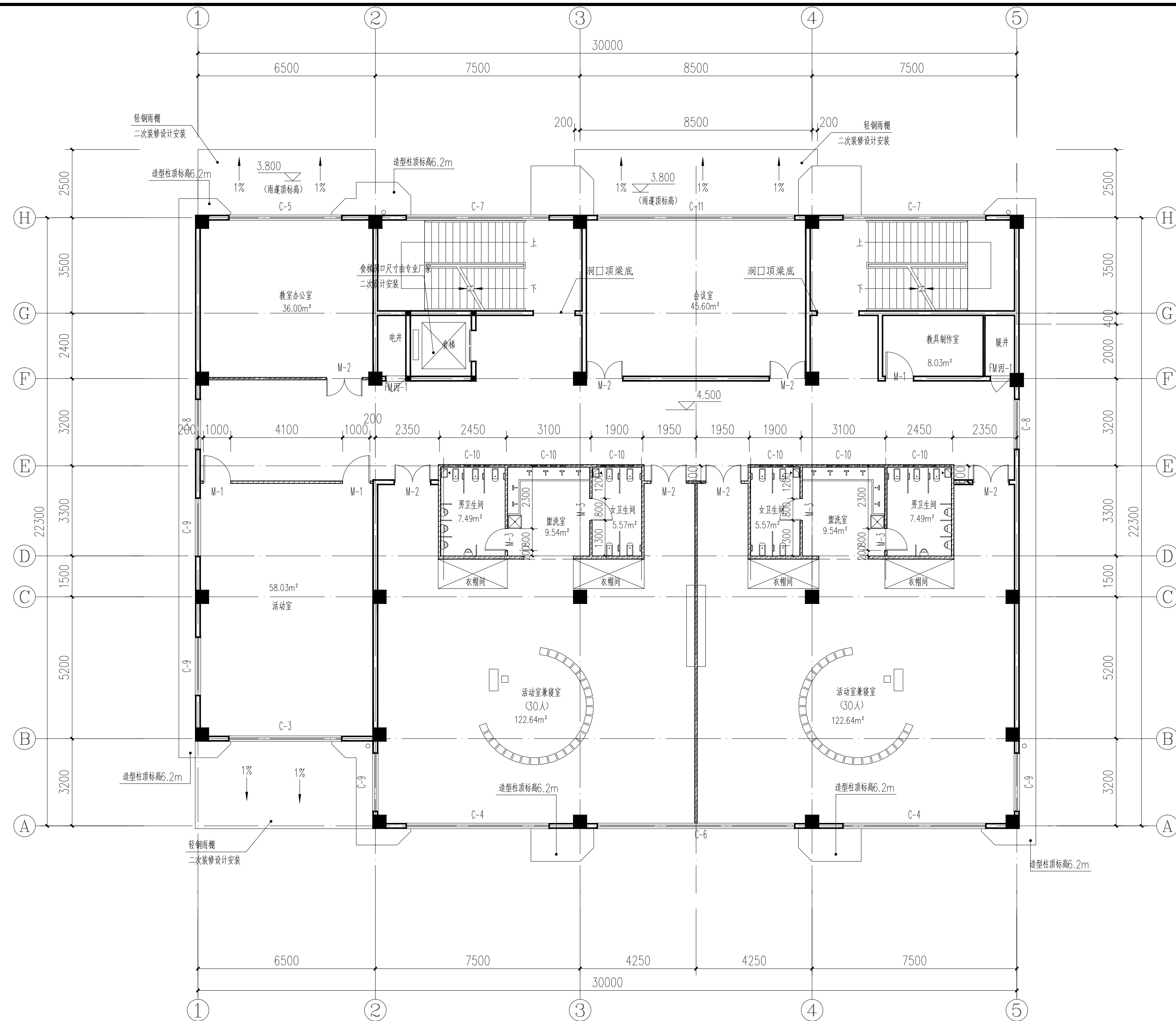
二层平面图 1:100
