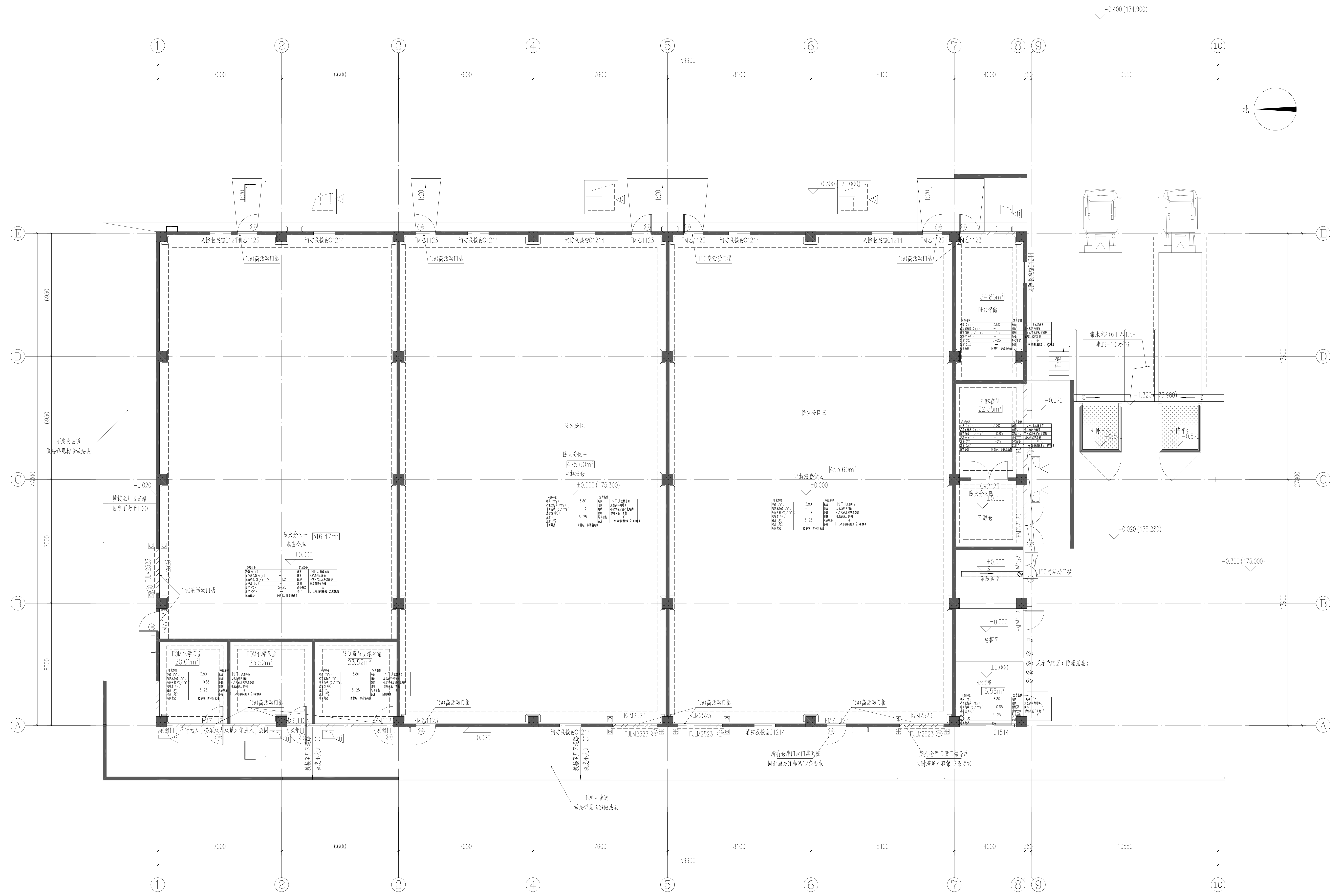
化学品仓1 首层平面图 1:100
