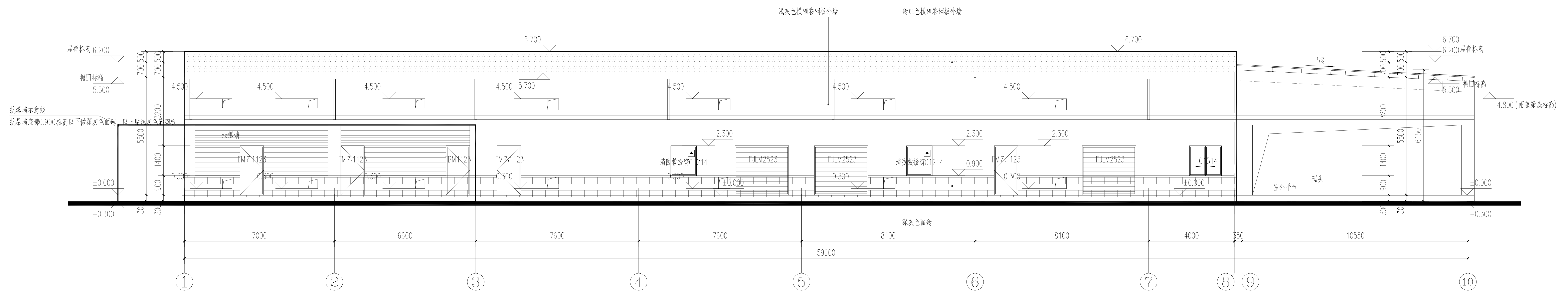
化学品仓1 ①轴~⑩轴立面图 1:100
