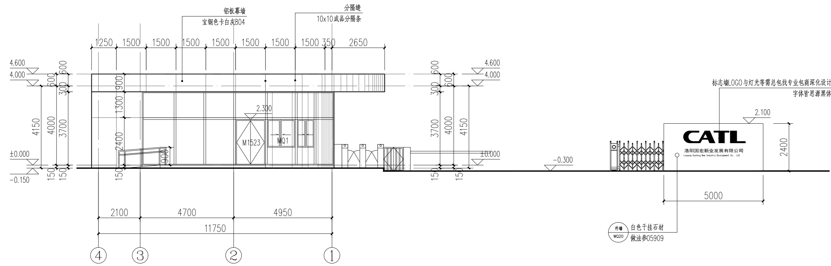
4-1轴立面图 1:100
