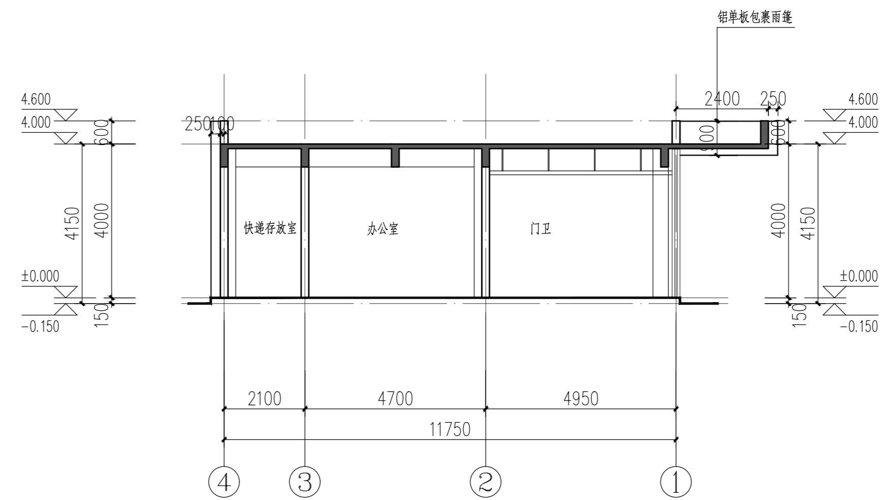
1-1轴剖面图 1:100
