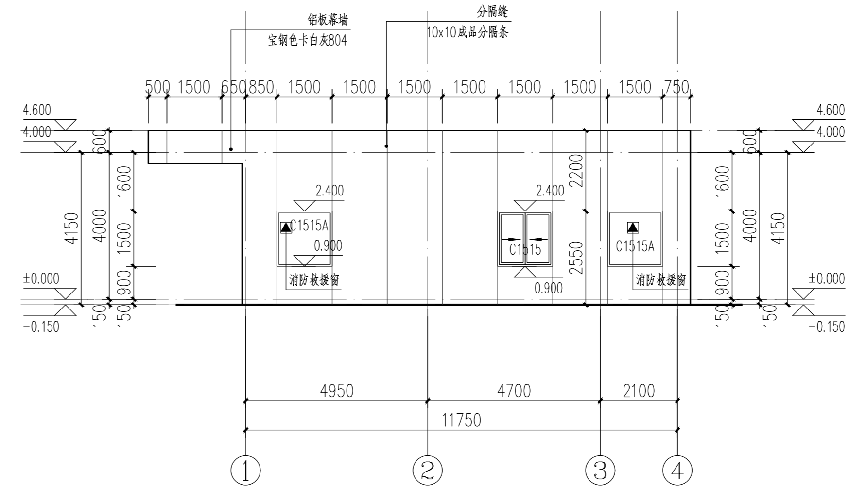
1-4轴立面图 1:100
