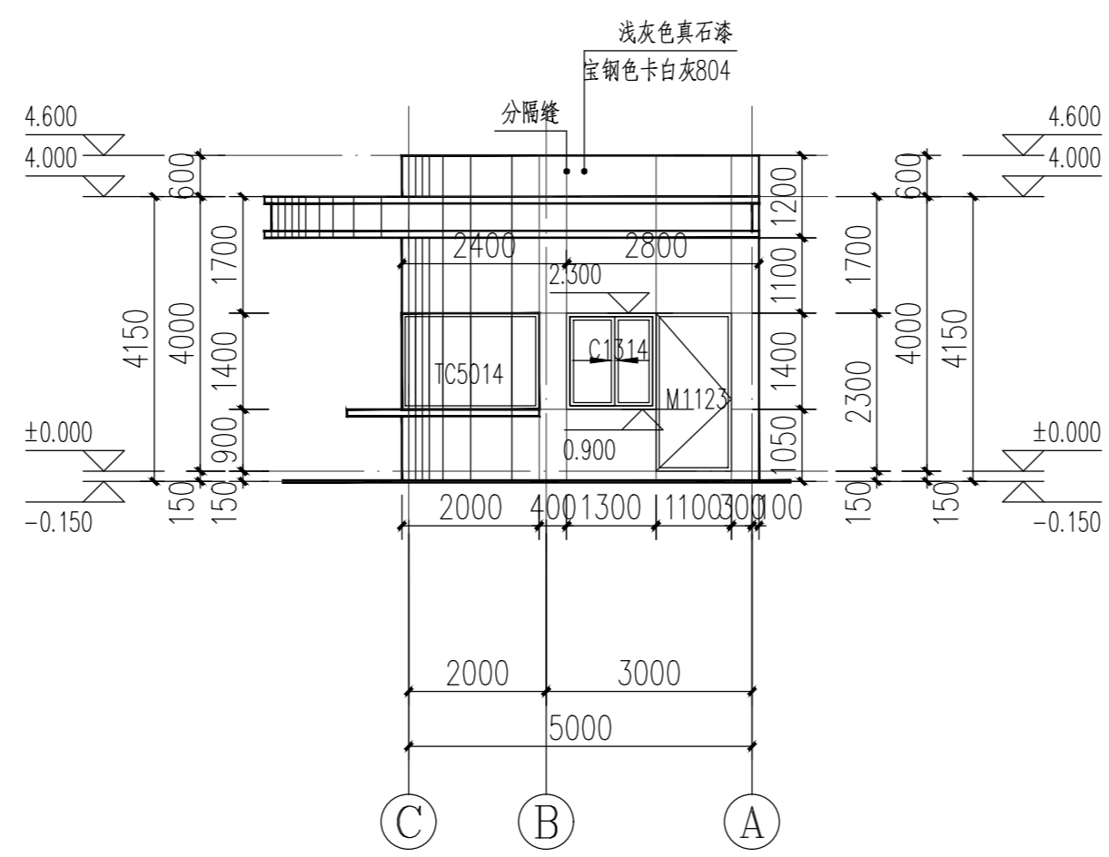
C-A轴立面图 1:100
