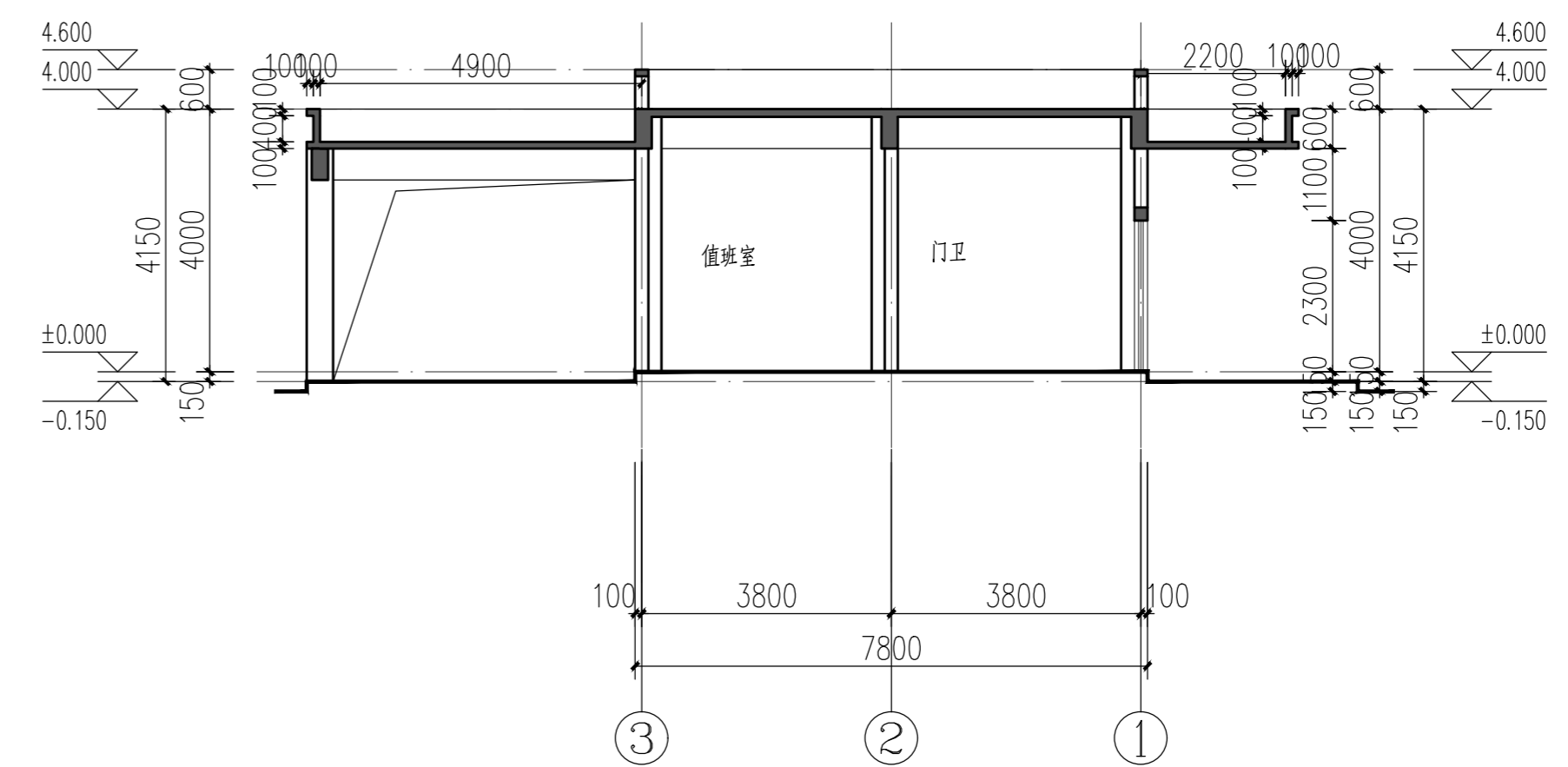
1-1剖面图 1:100
