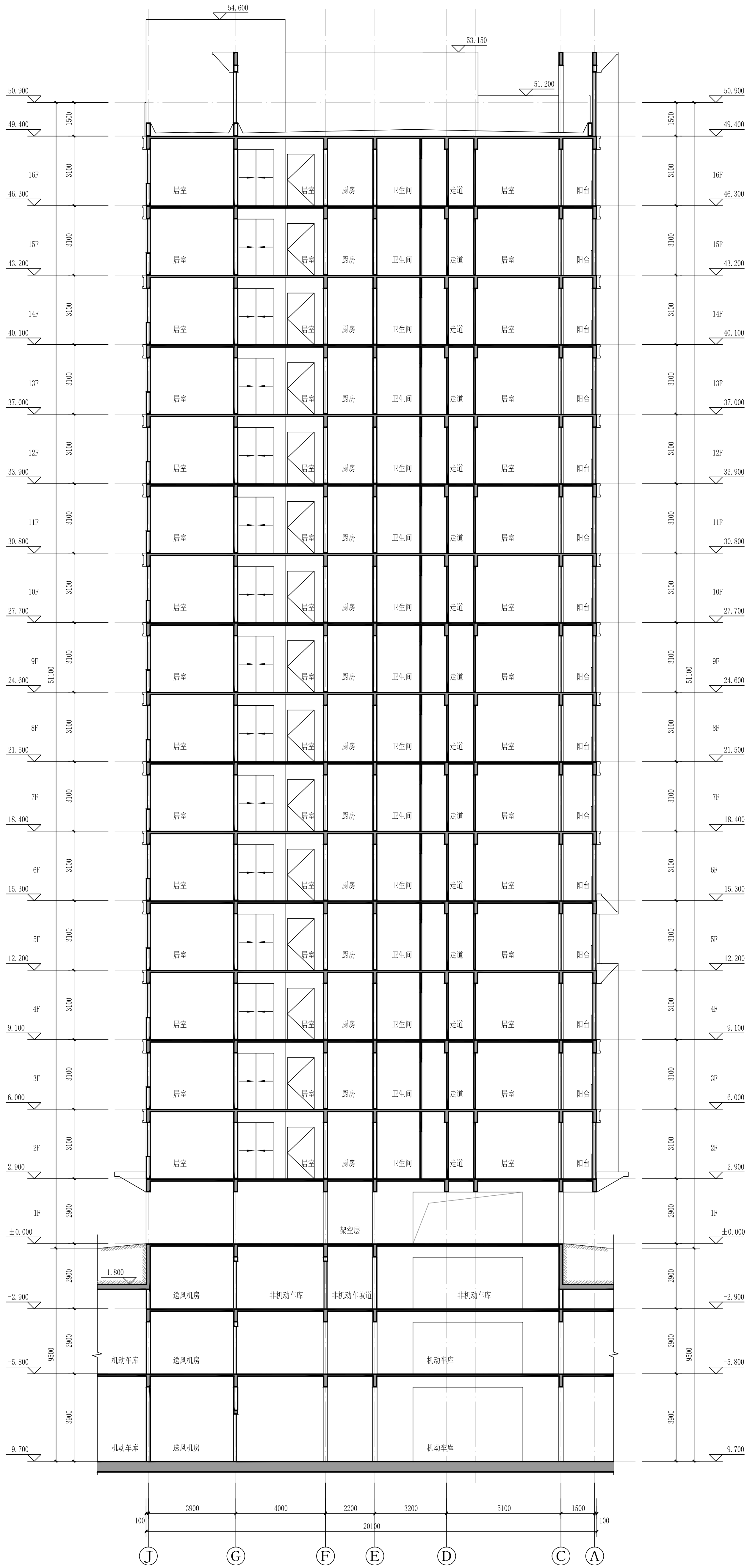
1-1剖面图 1:100
