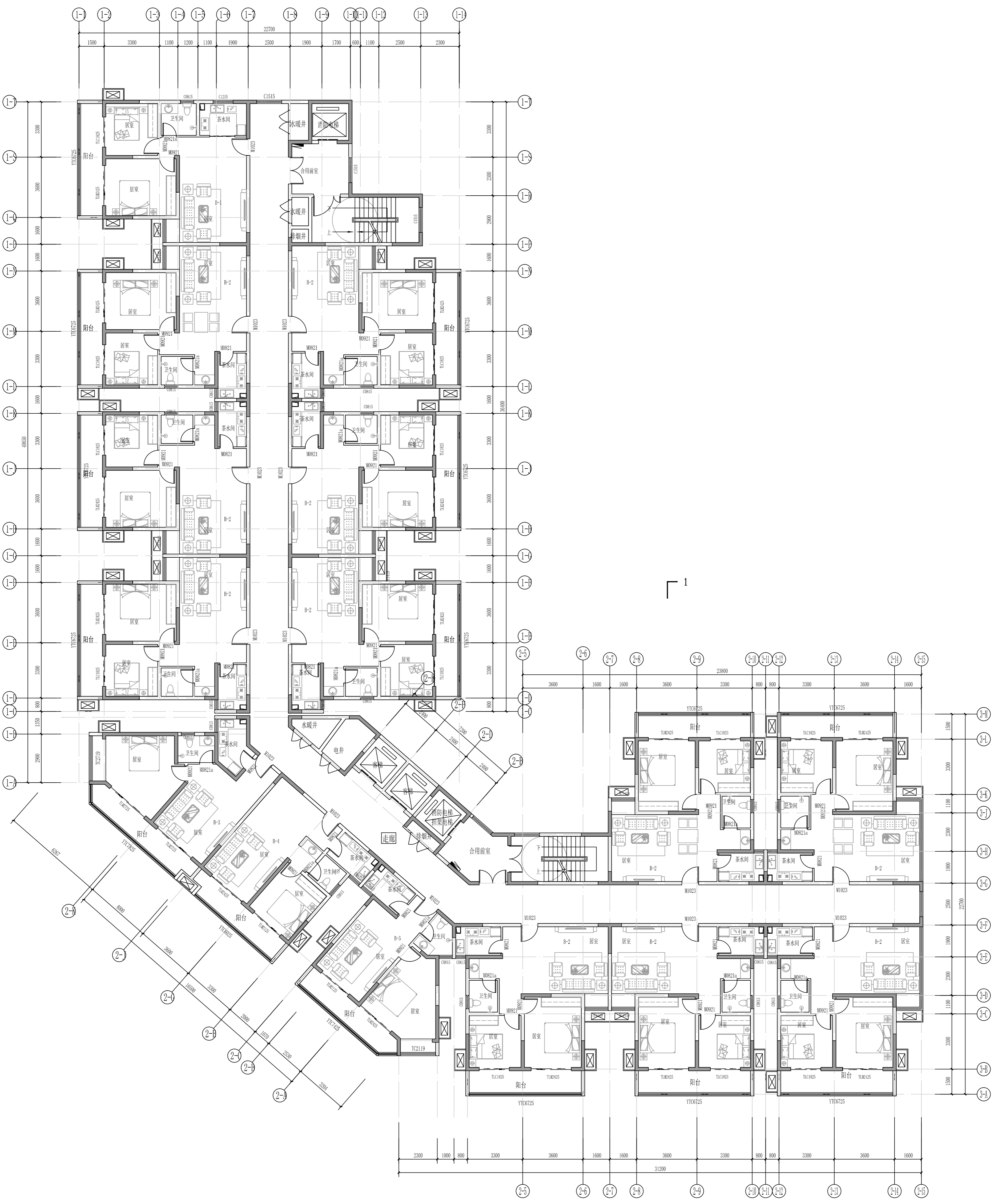
三-十六层平面图 1:100
