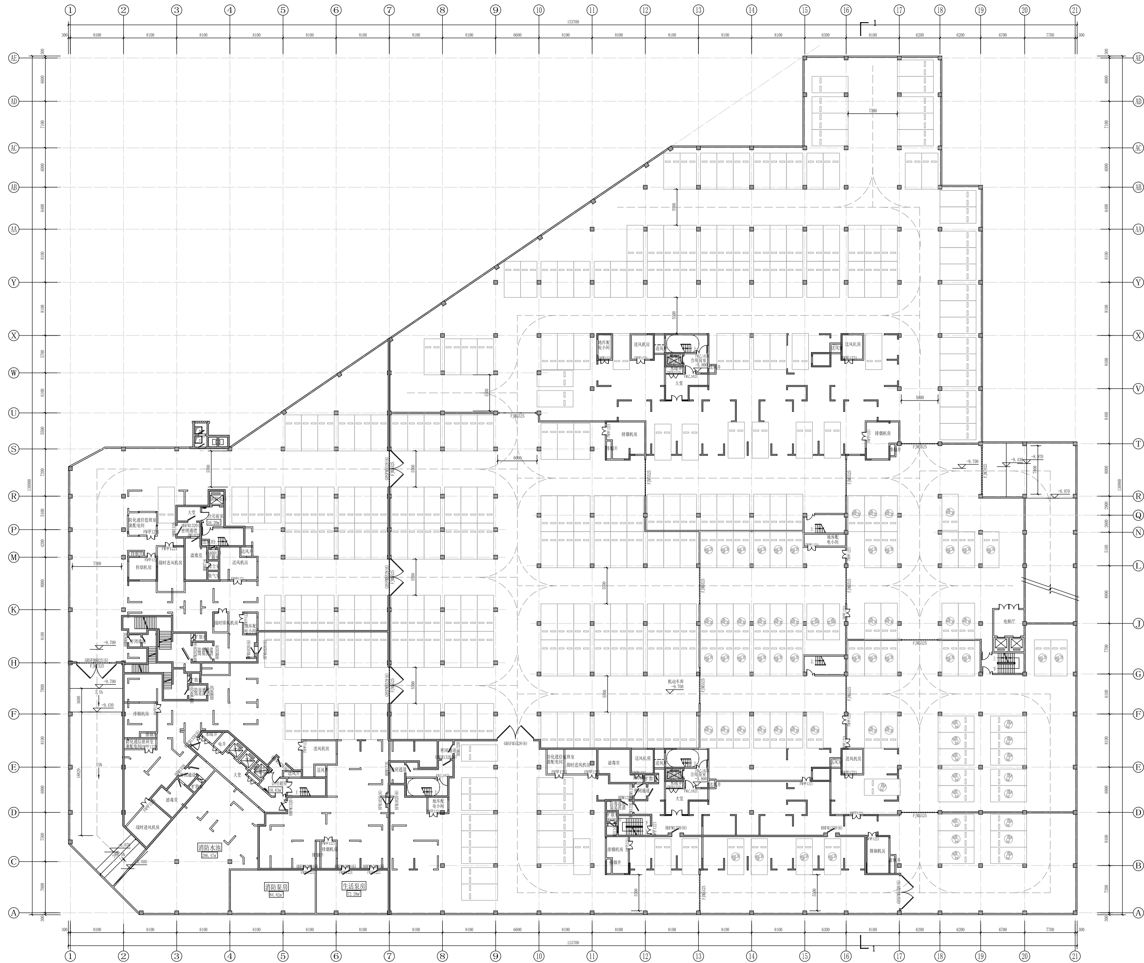
地下二层平面图 1:200
