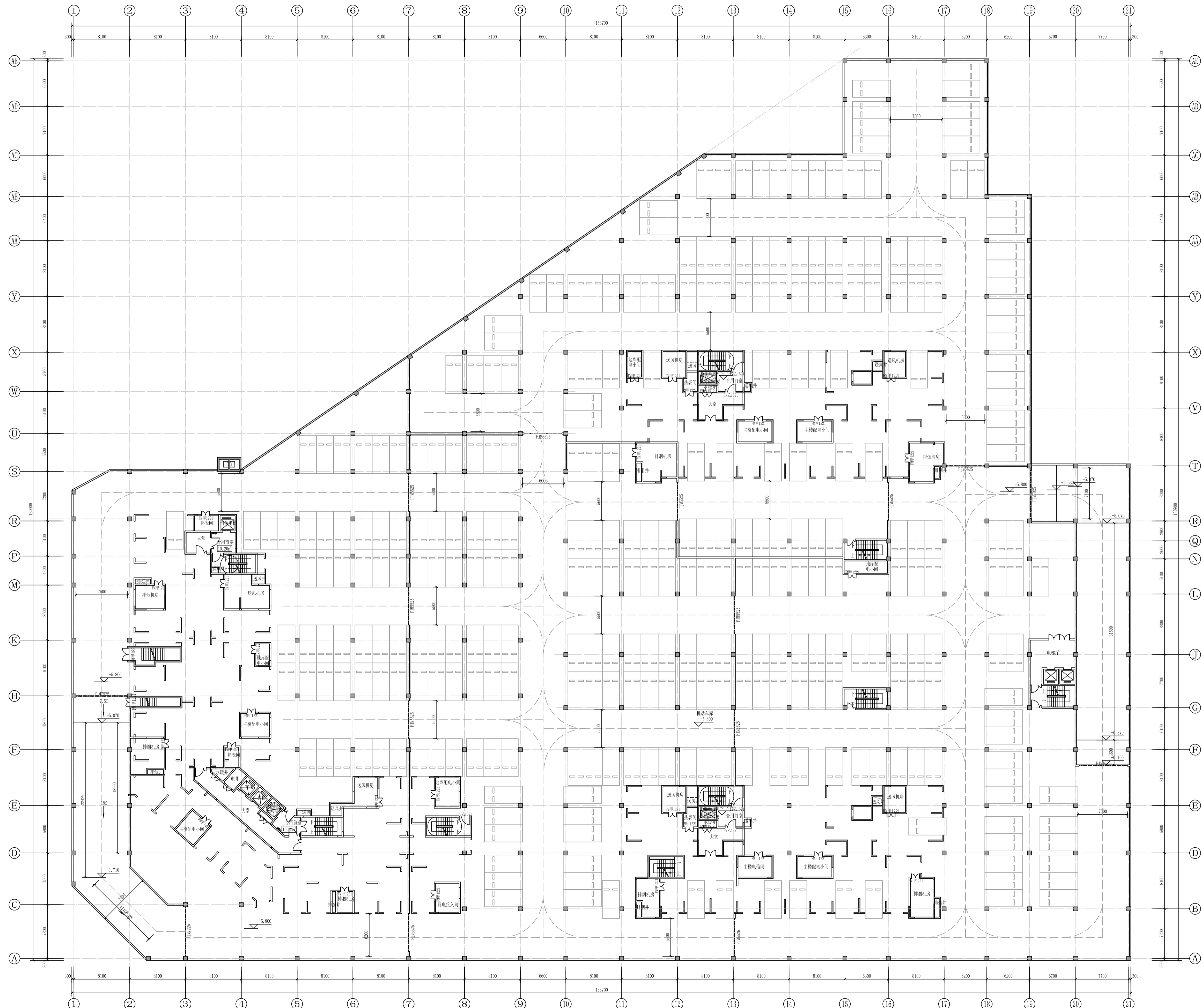
地下一层平面图 1:200
