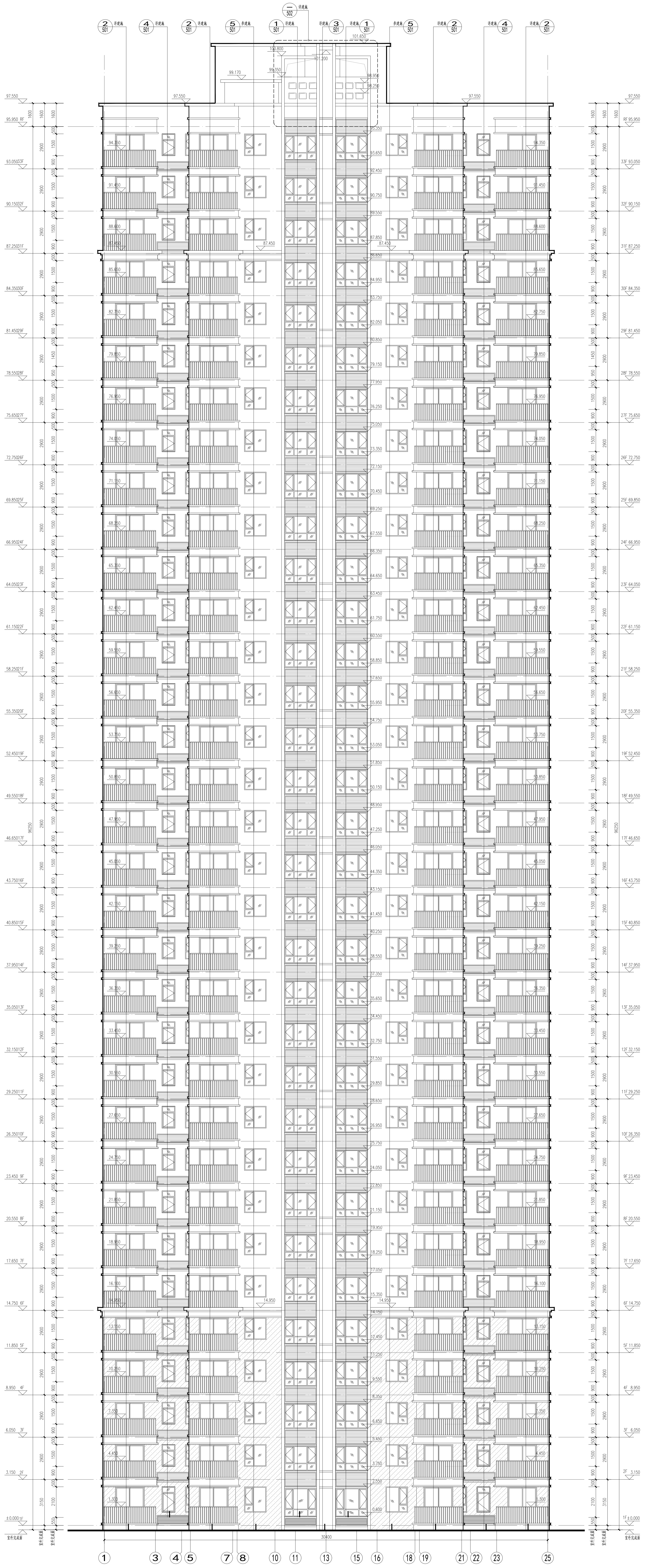
①-25立面图 1:100
