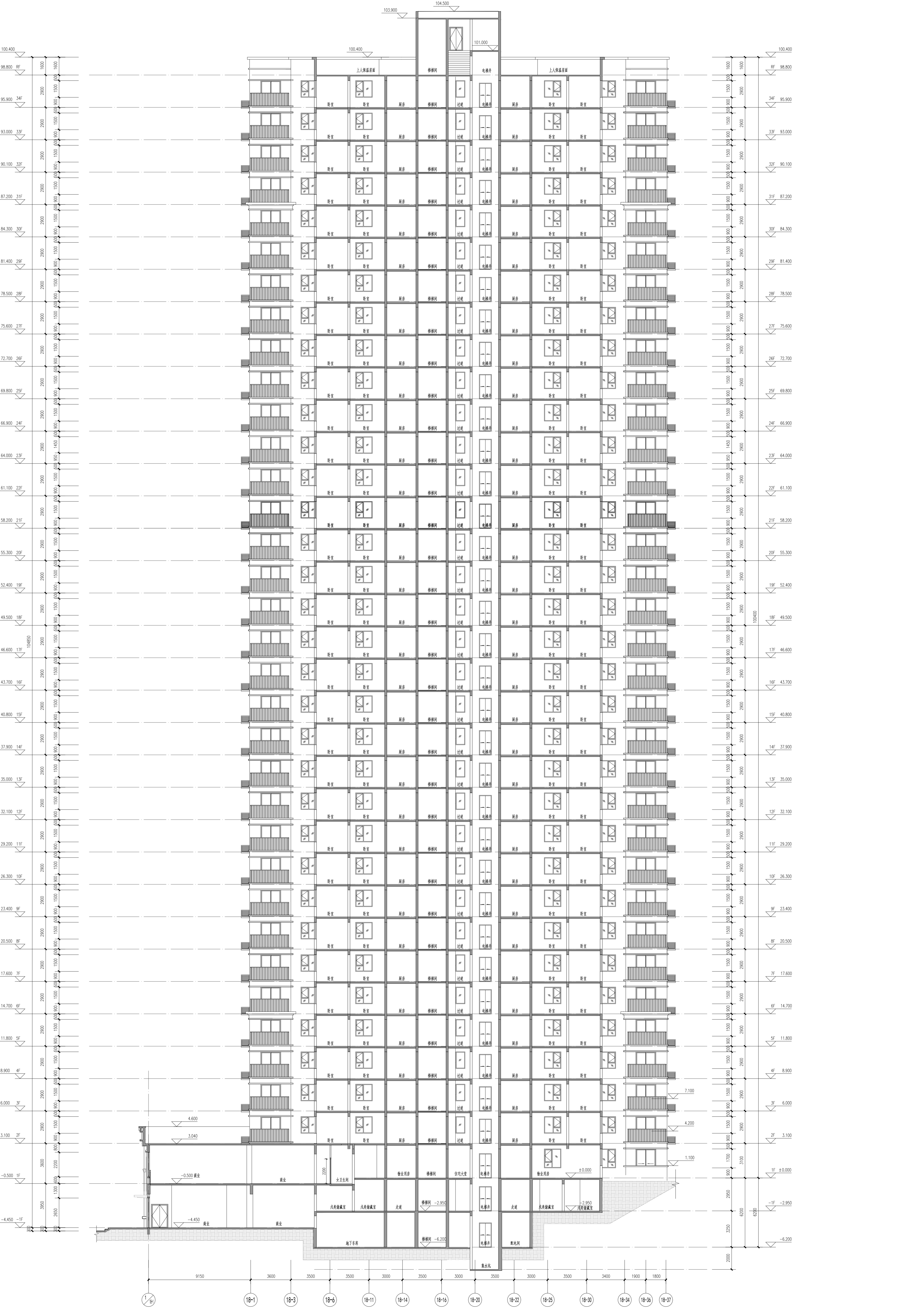
4-4剖面图 1:150
